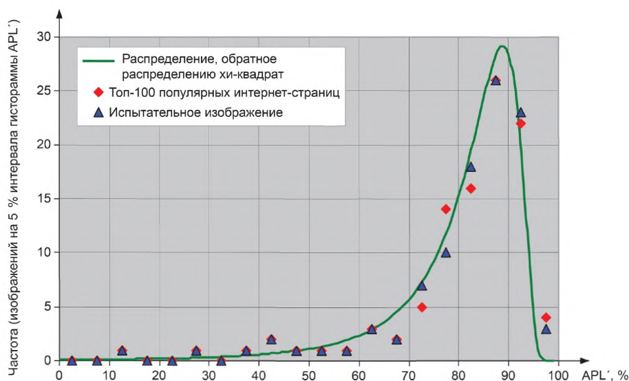
Рисунок А.2 — APL' видеосигнала с интернет-контентом
