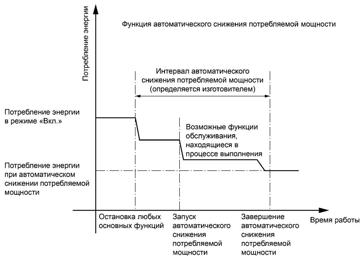
Рисунок 1 — Функция автоматического снижения потребляемой мощности
