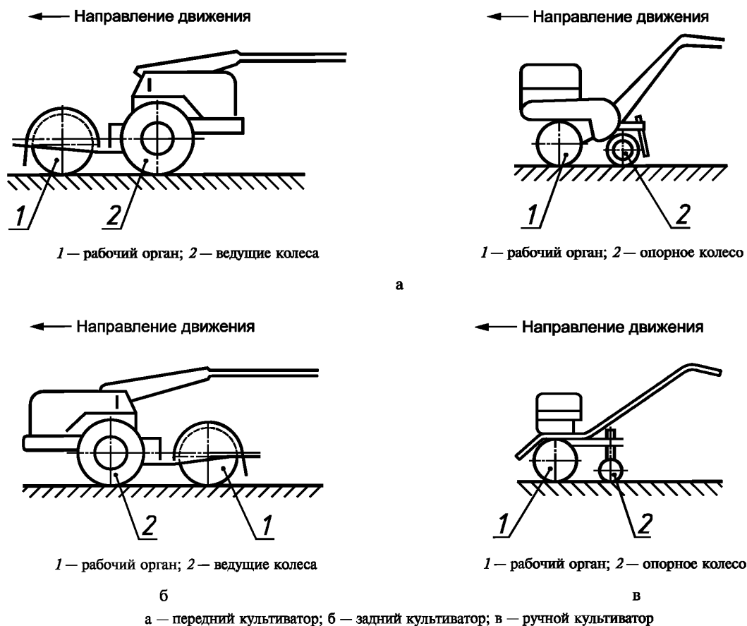
Рисунок 1 — Типы культиваторов
