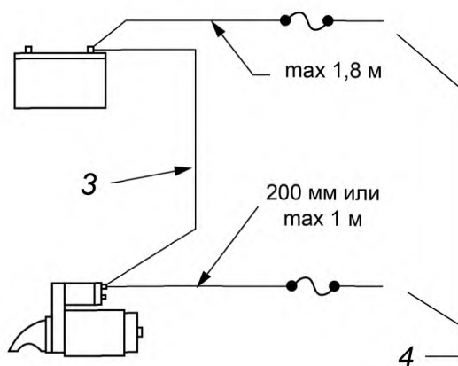
с) Без выключателя массы
