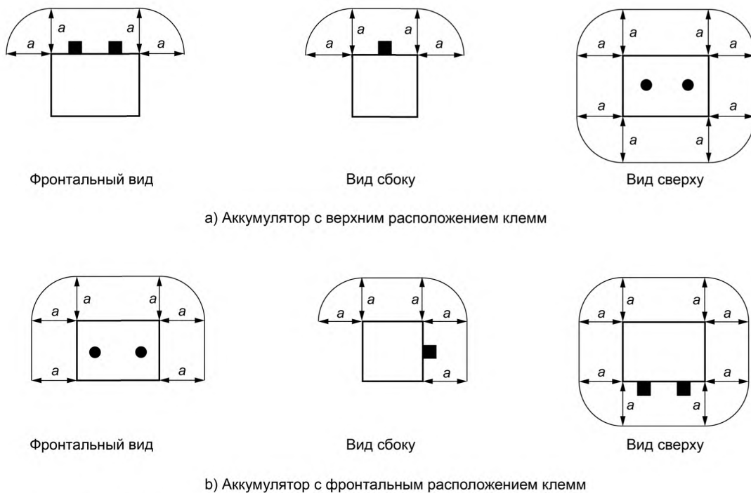
Рисунок 1 — Свободное пространство a вокруг аккумулятора
