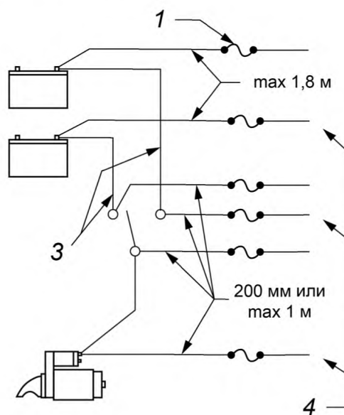
b) Двойной аккумулятор
