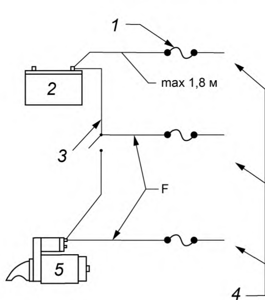
а) Одиарный аккумулятор
