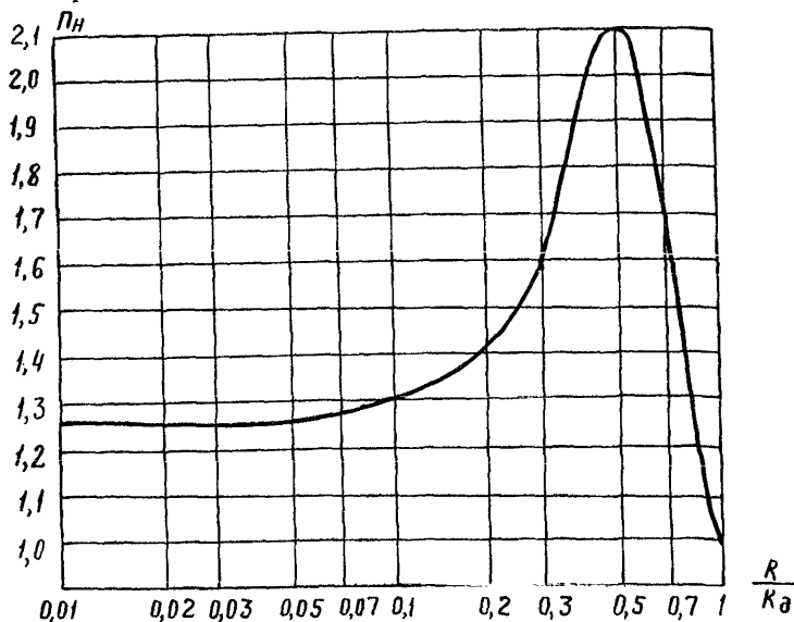
Рис. 2. Нормированная осевая ППЭ антенны с круглой апертурой. По — нормирована относительно значения По при R=R_d .
