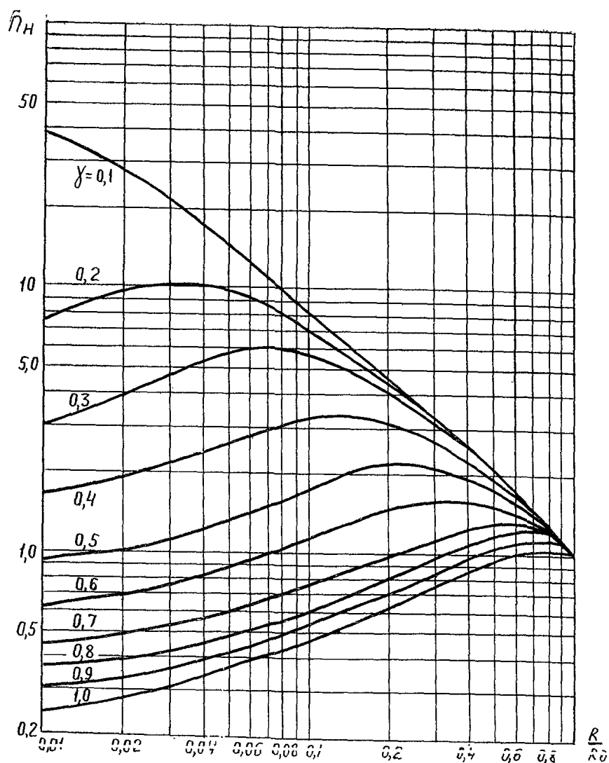
Рис. 1. Нормированная осевая ППЭ антенны с прямоугольной апертурой. \tilde{P}_H — нормирована относительно значения P_0 при R=R_d ; \gamma — соотношение вертикального и горизонтального размеров антенны.
