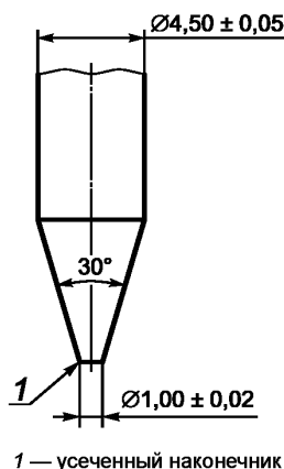
Рисунок 10 — Испытательный стержень для определения сопротивления проколу
