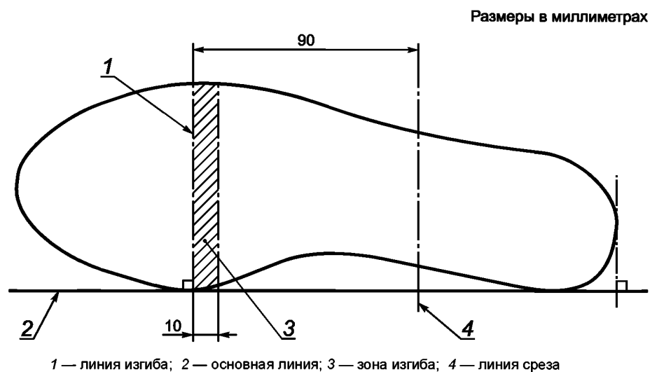
Рисунок 13 — Линия изгиба проколозащитных прокладок
