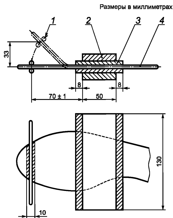
1 — направляющий стержень; 2 — прижимные пластины; 3 — резиновые пластины; 4 — испытуемый образец (проколозащитная прокладка)
