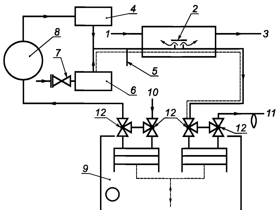
1 — линия подачи тест-вещества; 2 — адаптер для установки испытуемого образца клапана; 3 — сброс; 4 — абсорбер; 5 — линия отбора проб подаваемого воздуха; 6 — абсорбер; 7 — линия подачи воздуха с обратным клапаном; 8 — насытитель; 9 — искусственное легкое с двумя цилиндрами; 10 — линия подачи воздуха; 11 — линия отбора проб подаваемой газовой смеси; 12 — клапаны управления искусственным легким
