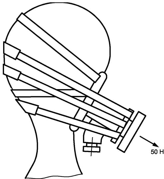
Рисунок 1 — Устройство для испытания соединительного элемента
