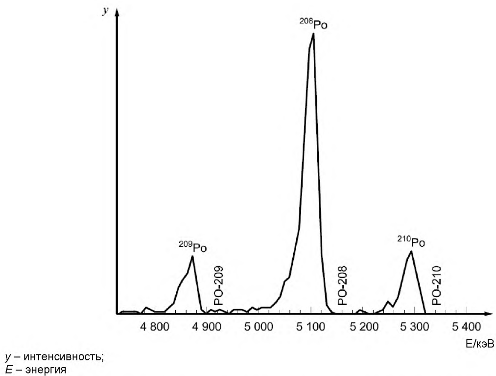
Рисунок В.2 – Пример спектра, полученного с использованием ионизационной камеры с сеткой с ^{208}\text{Po} в качестве трассера (метки)
