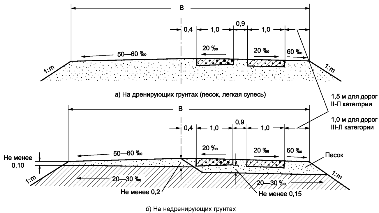
Рисунок В.2 — Для двухполосных лесных дорог
