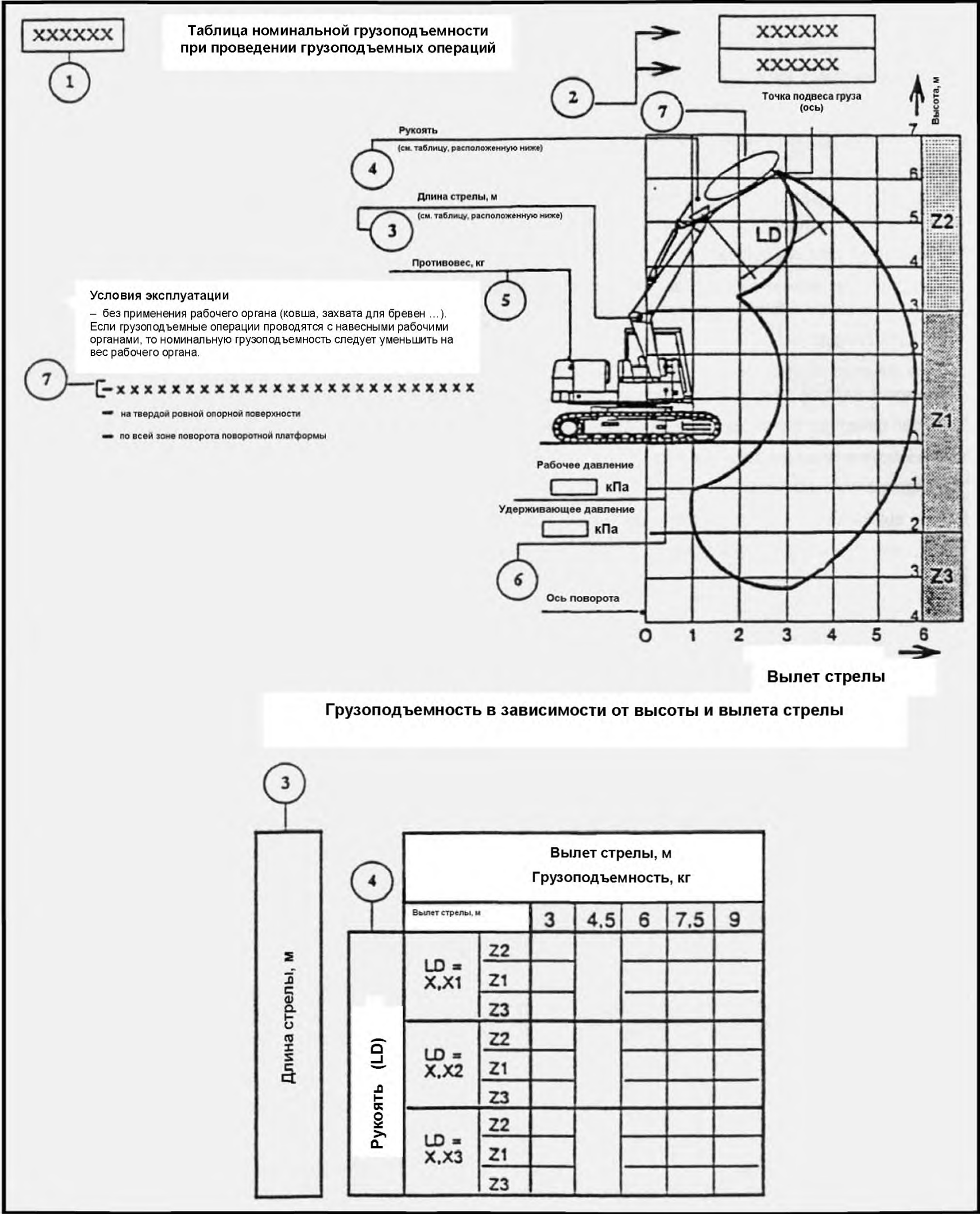
Т а б л и ц а В.1 – Таблица грузоподъемности для гусеничных экскаваторов
