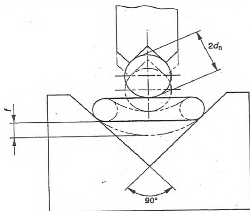
Рисунок 2 – Прогиб f
