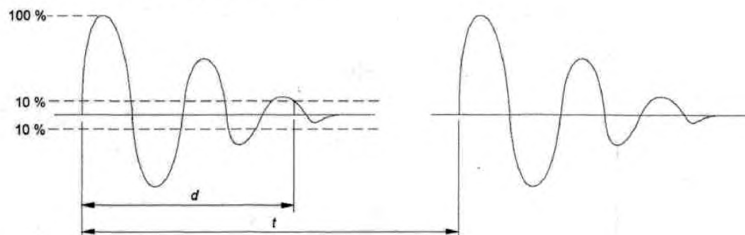
Рисунок 101 — Форма импульса
