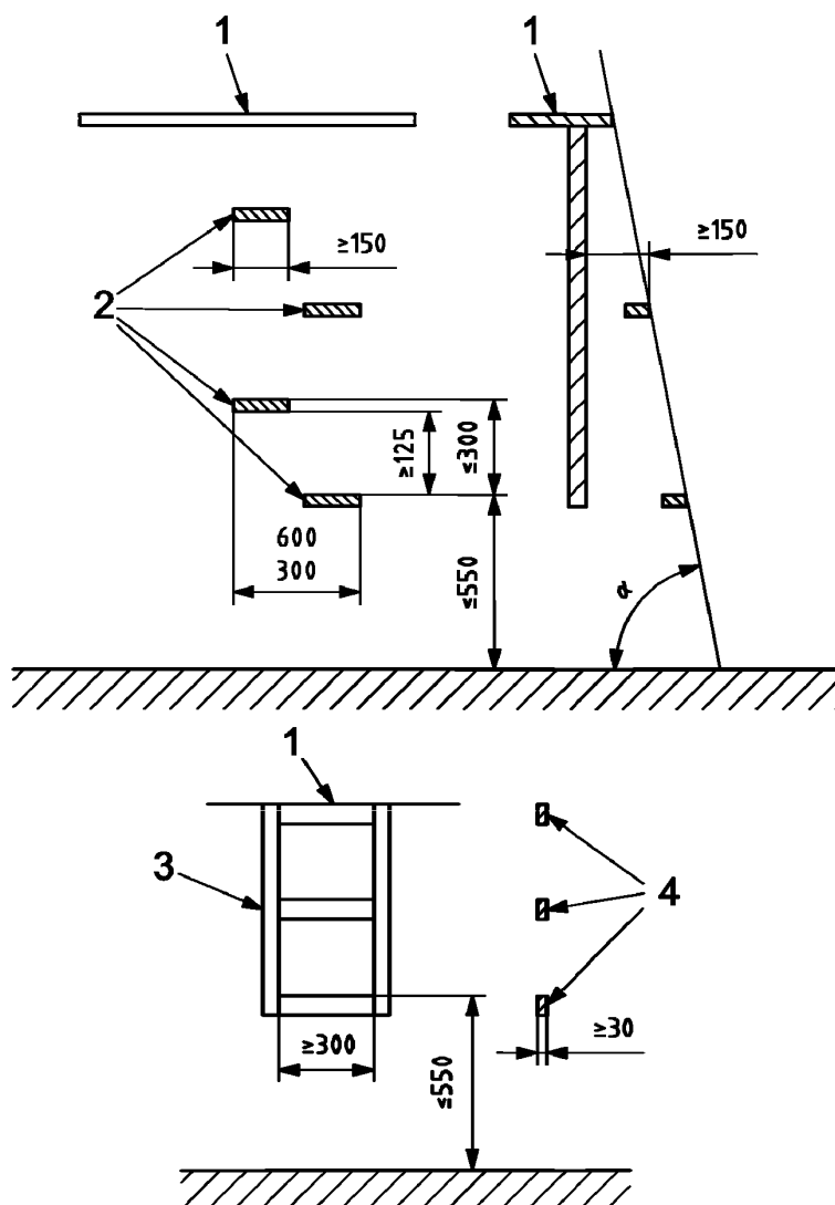
1 – платформа; 2 – ступень; 3 – лестница; 4 – перекладина
