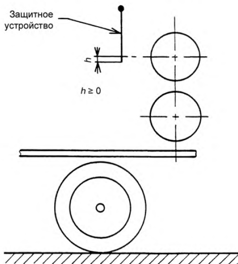
Рисунок 1 – Защитное устройство
