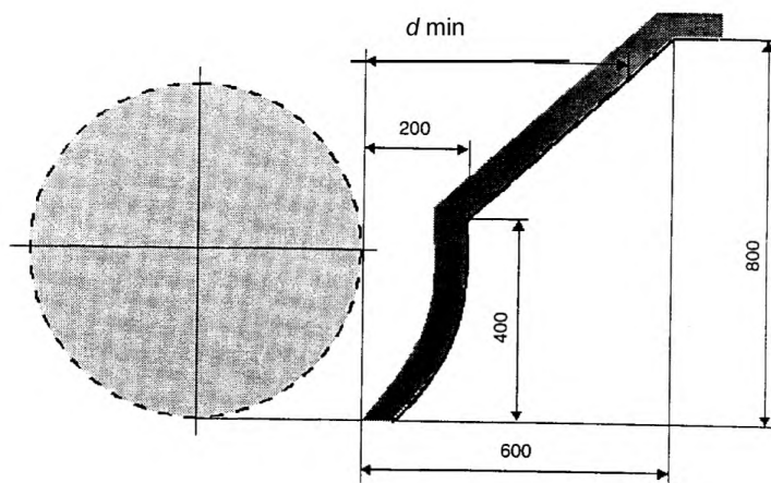
Рисунок 4 – Заднее защитное ограждение с шарниром
