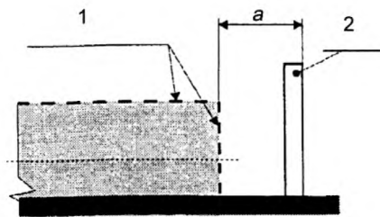
1 – траектория движения рабочего органа; 2 – защитное ограждение
