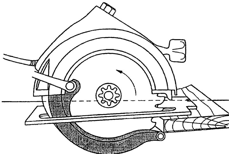
Рисунок 4 – Пример автоматически запирающегося съемного защитного устройства
