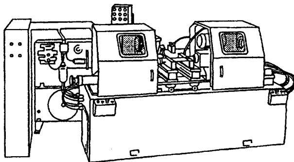
Рисунок 7 – Пример блокируемых подвижных съёмных защитных устройств
