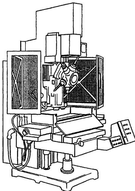
Рисунок 6 – Пример съёмных защитных устройств, блокируемых откидными ограждениями
