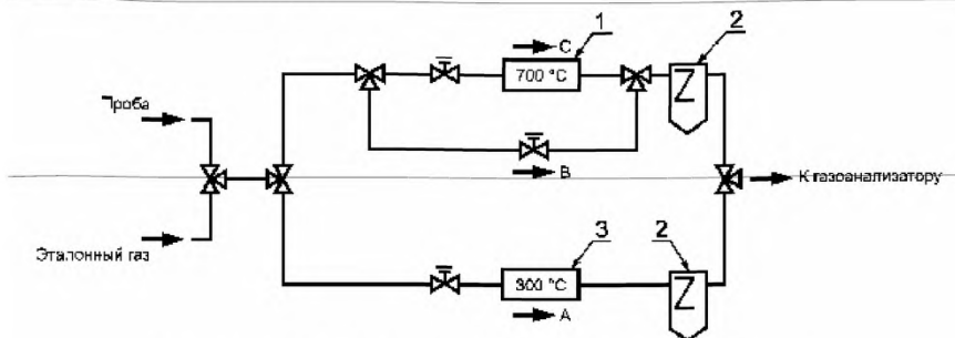
1 — конвертер; 2 — влагоотделитель с холодильником; 3 — конвертер из графита, А — измерение концентрации NO x ; В — измерение концентрации NO; С — измерение концентрации NO x + NH 3 . Концентрация NO 2 равна А — В. Концентрация NO 3 равна С — А. Рисунок 2 — Схема измерения концентрации NH 3
