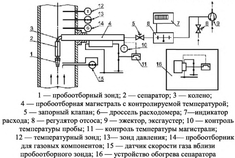
Рисунок 4 — Система измерения весовой концентрации твердых частиц (с внутренним сепаратором)
