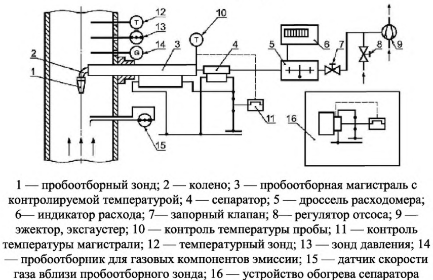
Рисунок 5 — Система измерения весовой концентрации твердых частиц (с внешним сепаратором)
