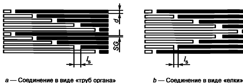
Рисунок 2 — Части типичных простых четырехступенчатых соединений
