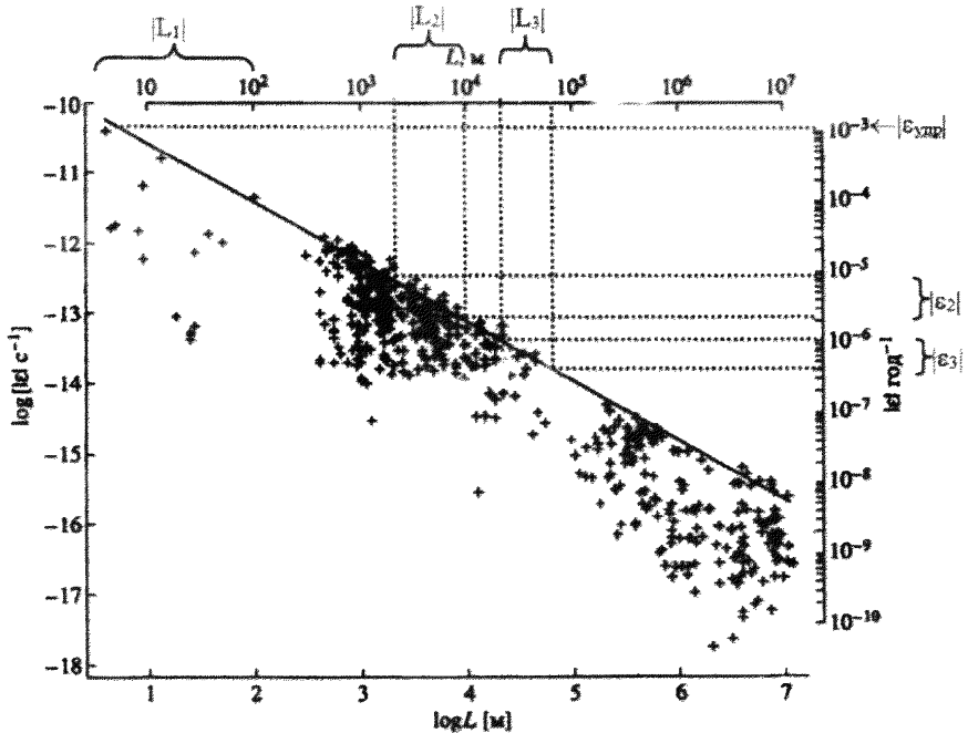
Рис. 1. Распределение модулей скоростей предельных горизонтальных деформаций в зависимости от расстояния между пунктами наблюдений
