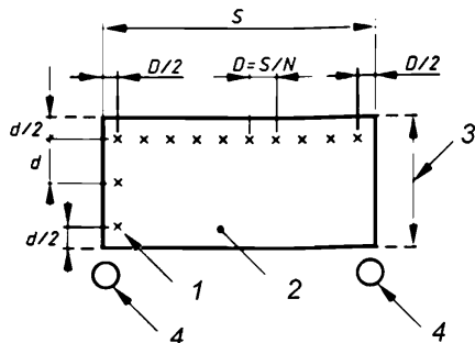
Рисунок 6.4 – Расчетное поле для расчета освещенности
