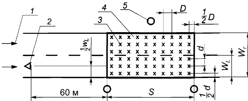
Рисунок 6.9 – Примеры расчетных полей
