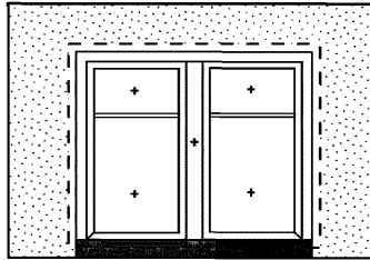
Рисунок 6.8 – Пример расположения контрольных точек для расчета E_v
