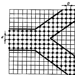
Рисунок 6.5 – Выбор расчетных точек на нестандартном расчетном поле
