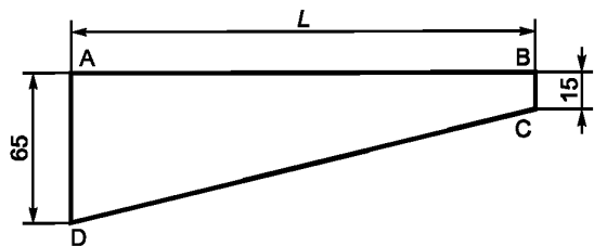
Рисунок 2 — Образец для испытаний типа 2 (клиновидный)
