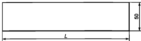
Рисунок 1 — Образец для испытаний типа 1 (прямоугольный)
