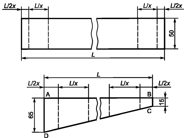
Рисунок 3 — Точки измерения
