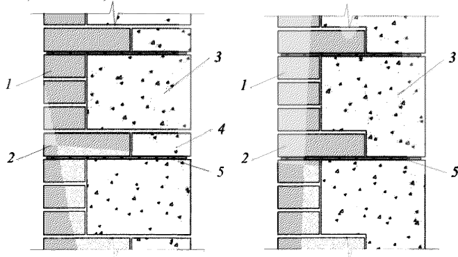
а) Двухслойные стены с горизонтальными рядами
