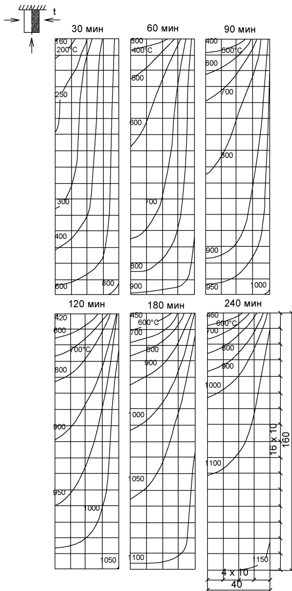
Рисунок И.5 - Балка из тяжелого бетона сечением 160х80 мм при нагреве с трех сторон
