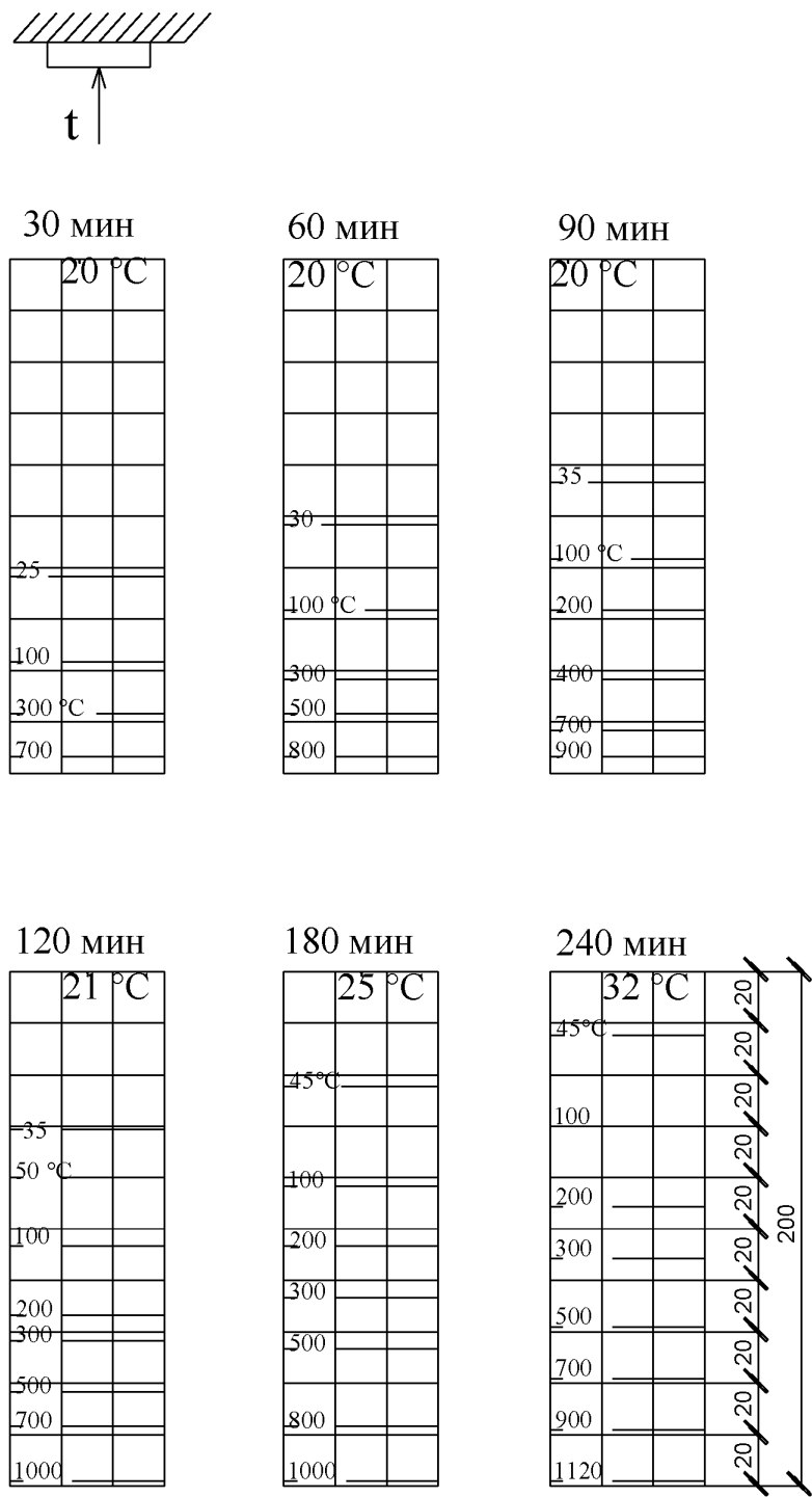
Рисунок И.15 - Плита из легкого бетона толщиной 200 мм при нагреве с одной стороны
