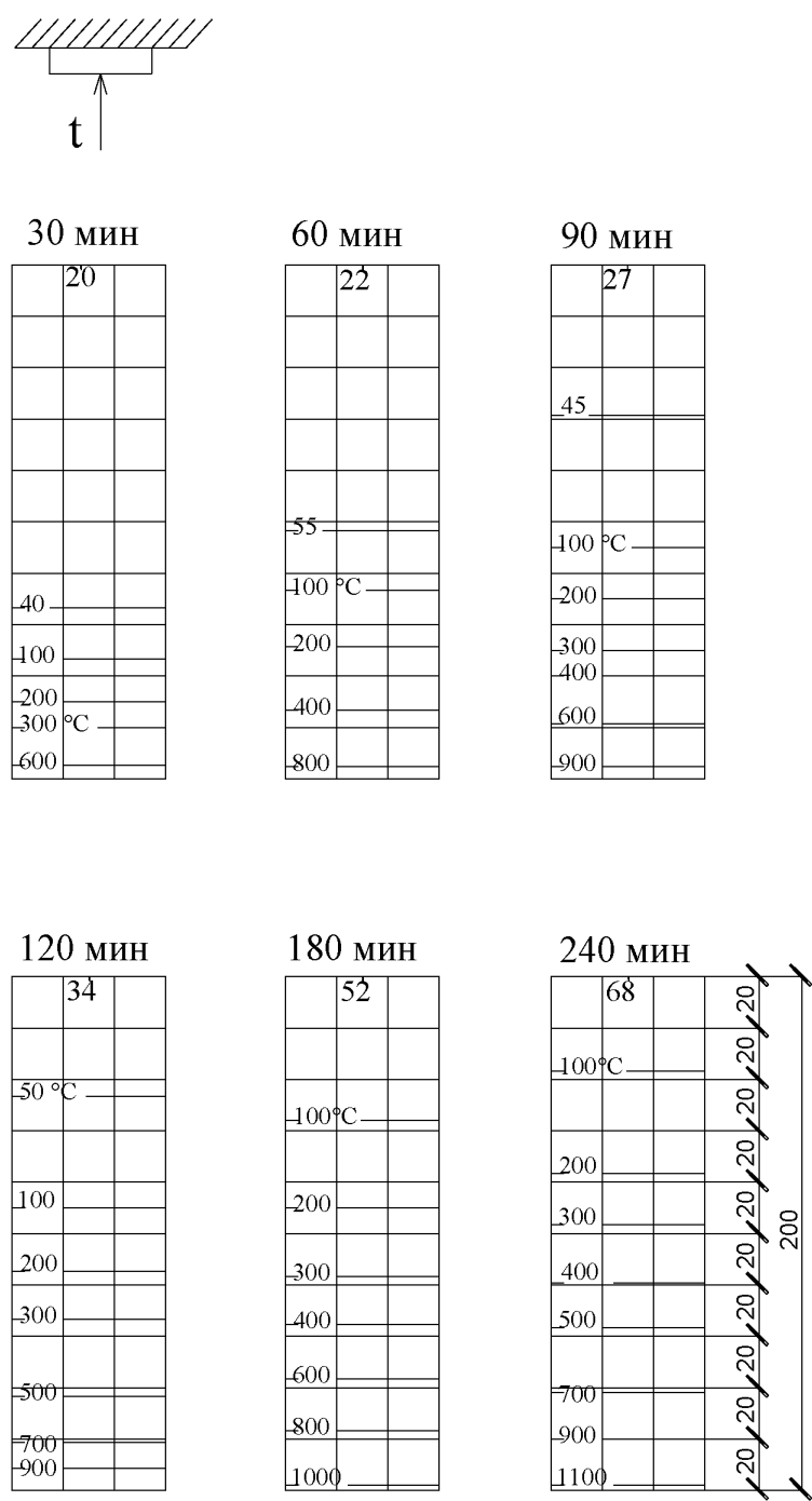
Рисунок И.12 - Плита из тяжелого бетона толщиной 200 мм при нагреве с одной стороны
