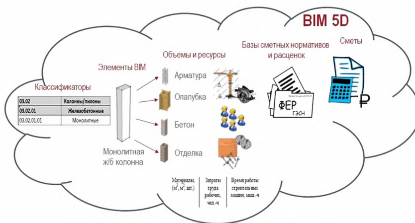
Рисунок 7.3 – Элементы информационной модели 5D
