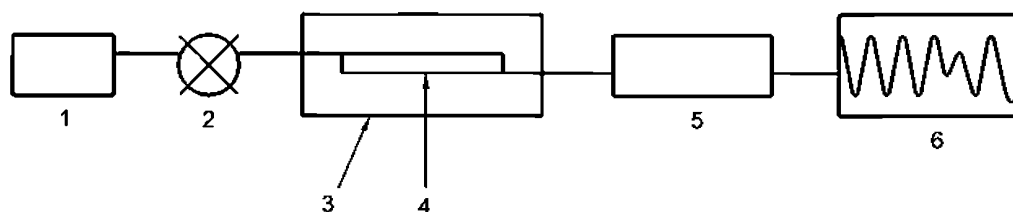
1 – насос; 2 – устройство ввода; 3 – термостат; 4 – колонка; 5 – рефрактометрический детектор; 6 – система обработки данных
