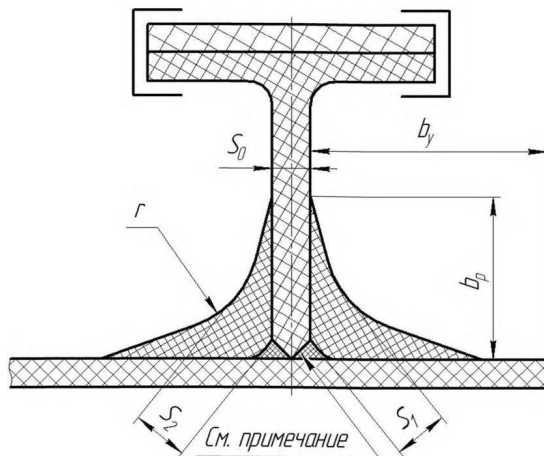
Рис. 5.5.4: b_y \geq 7S_0 > 30 мм; S_1 \geq 1/8b_y ; S_2 = 1/4b_y ; r = S_2
