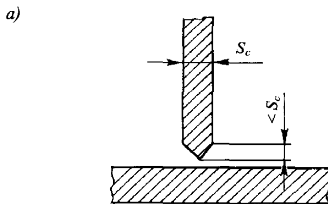
Рис. 5.3.1-2: S = (1/8 + 1/3)h ; h \geq 50 мм
