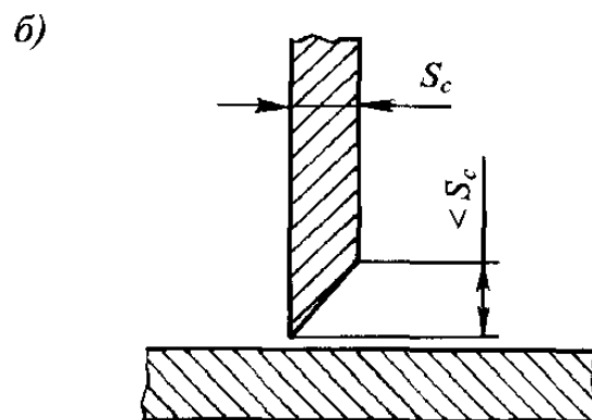
Рис. 5.3.2: а) — S_c \geq 10 мм; б) — 10 \geq S_c > 3 мм
