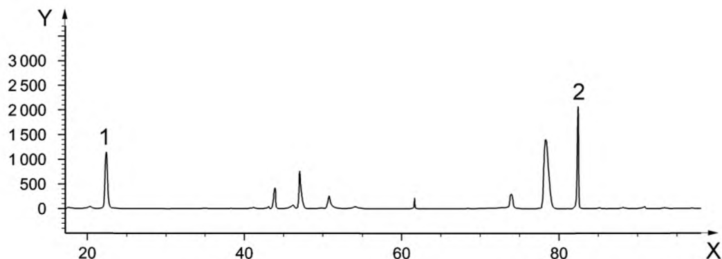
а) Хроматограмма разделения спирто-эфирной смеси при температуре 125 °С
