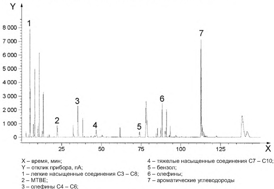
Рисунок В.1 – Типовая хроматограмма автомобильного бензина, содержащего МТВЕ
