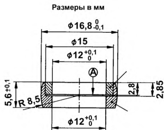
Рисунок 7 – Фильтрующее устройство
