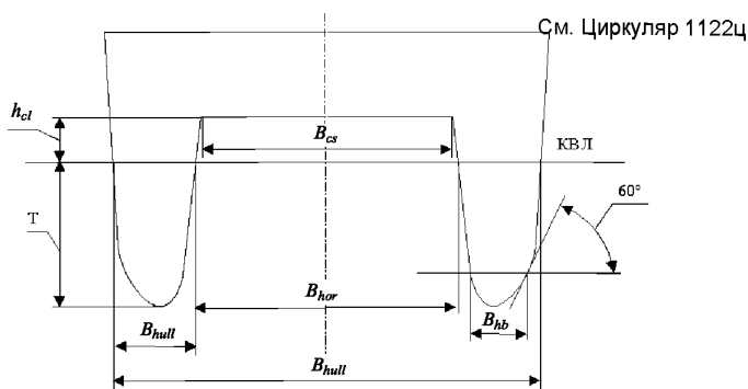
Конструктивные параметры катамарана
