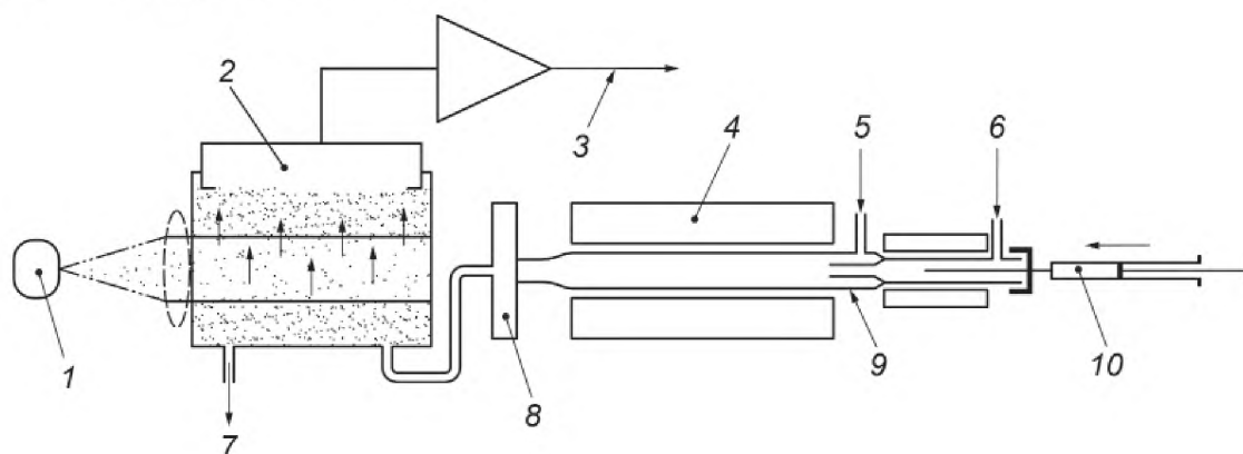
1 — источник УФ-излучения; 2 — фотоумножитель; 3 — выходной сигнал; 4 — печь, обеспечивающая температуру 1000—1100 °С; 5 — устройство подачи кислорода; 6 — устройство подачи инертного газа; 7 — газотвод; 8 — осушительная камера паров; 9 — кварцевая камера; 10 — микрошприц
