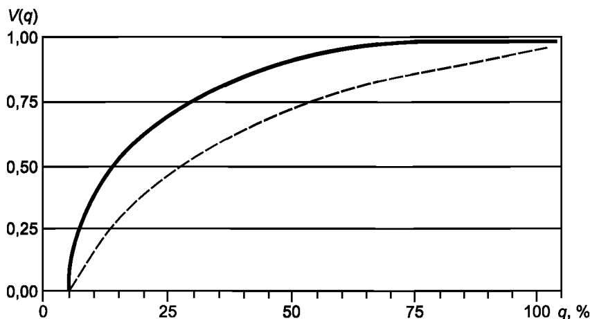
V(q) — выявляемость, q — дефектность, \alpha — вероятность перебраковки, — — — — контроль по методике с вероятностью перебраковки \alpha = 0,05 , — — — — контроль по методике с вероятностью перебраковки \alpha = 0,15 .
