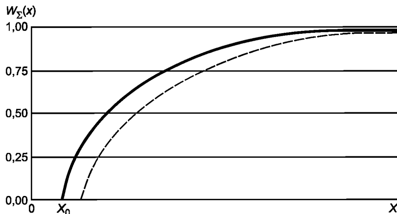
W_{\Sigma}(x) — суммарная выявляемость дефектов, X — размер (характеристический размер) дефекта, X_0 — размер наименьшего выявляемого дефекта, — — — кривая средних значений суммарной выявляемости, — — — — нижний 95 %-ный уровень доверительной вероятности.
