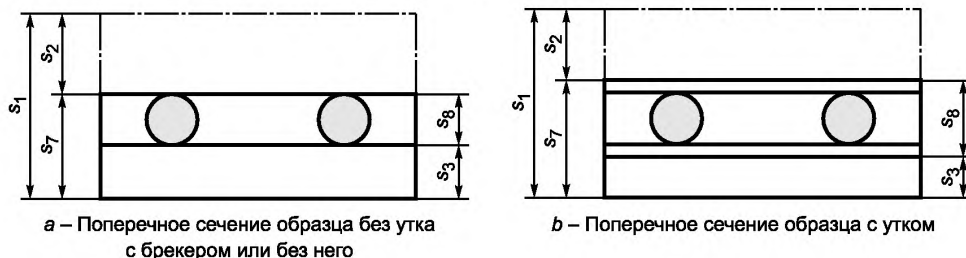
Рисунок 3 — Образцы для метода A1
