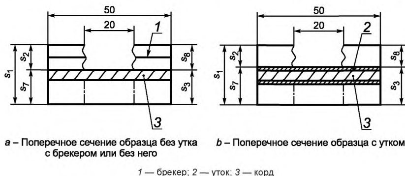
Рисунок 4 — Испытуемые образцы для метода A2
