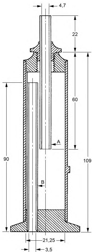
Рисунок А.1.2 — Резервуар
