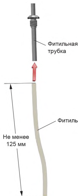
Рисунок 3 — Фитильная трубка
