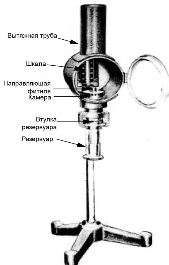
Рисунок 1 — Лампа для определения максимальной высоты некопящего пламени (ручной аппарат)
