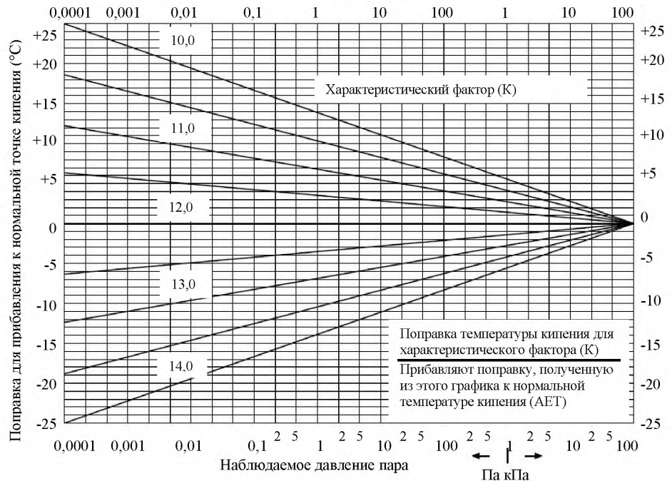
Рисунок Ж.2 – Поправки температур кипения для К-фактора
