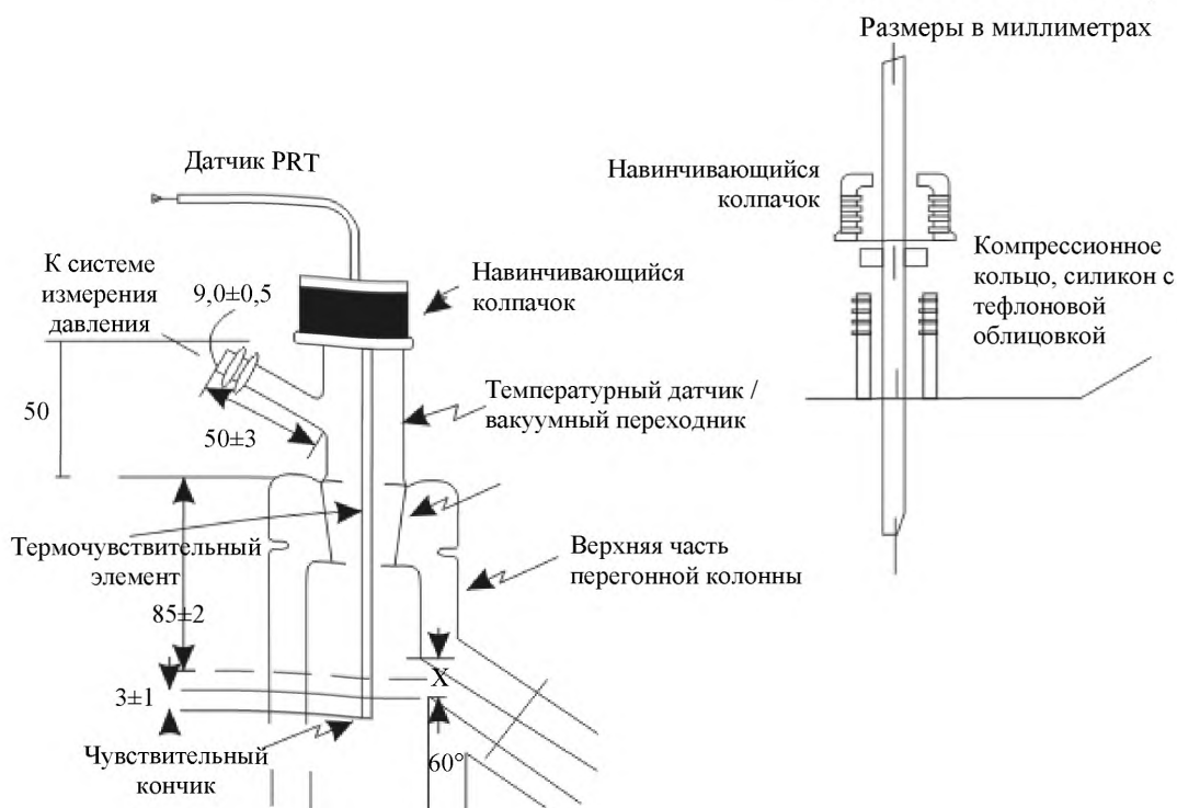
Рисунок 6 – Размещение температурного датчика
