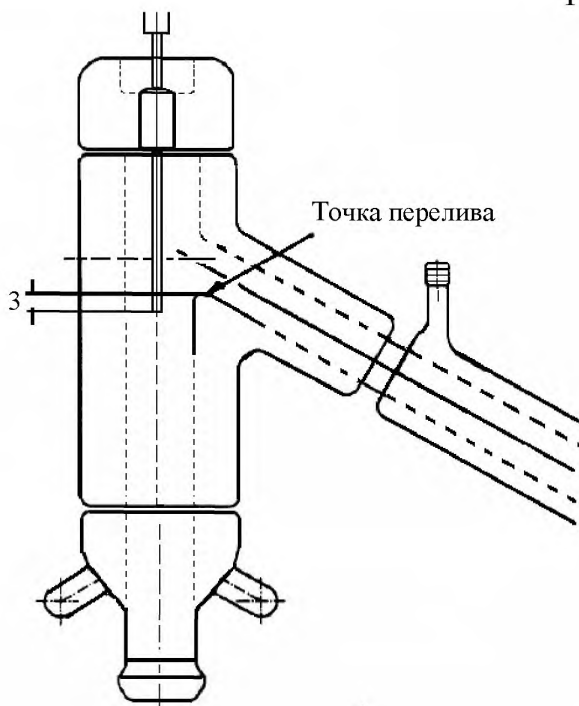
Рисунок 8 – Термопара
