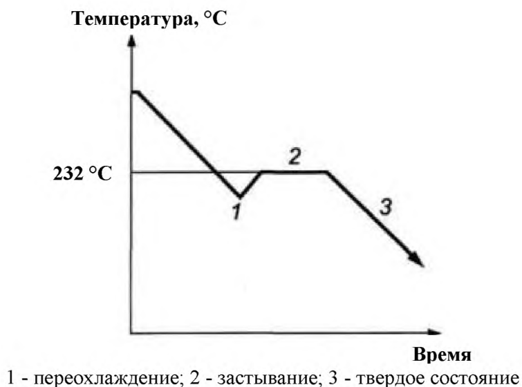
Рисунок A2.5 - Характеристики застывания олова
