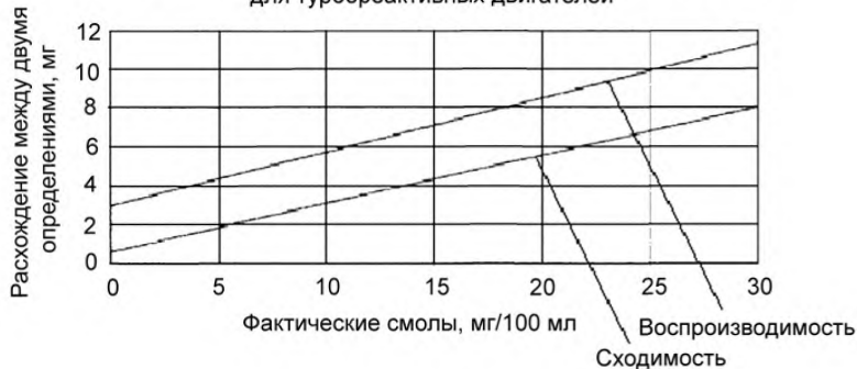
Рисунок 2 – Точность определения содержания фактических смол
