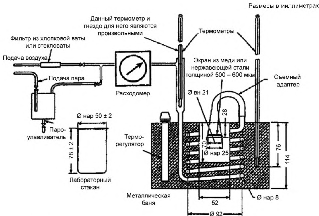
Рисунок 1 – Аппарат для определения содержания смол методом выпаривания струей
