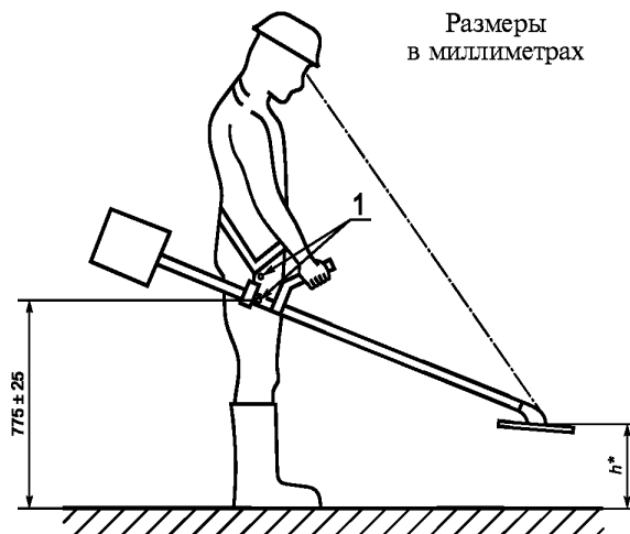
Рисунок 2 — Положение машины при испытании
