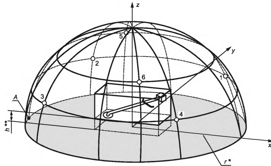
* Радиус полусферы r = 4 м. ** h = 300 мм для кусторезов и 50 мм для мотокоз. 1, 2, 3, 4, 5, 6 — микрофоны
