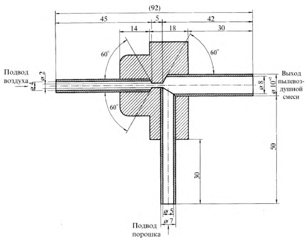
Рисунок 3 – Инжектор порошка
