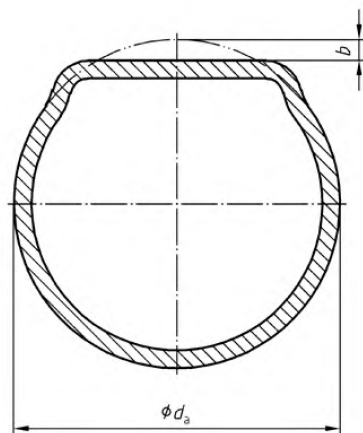
Рисунок Е.3 – Уплотнение цилиндрических обечайек
