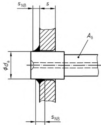
Рисунок D.12 – Вварной анкерный болт
