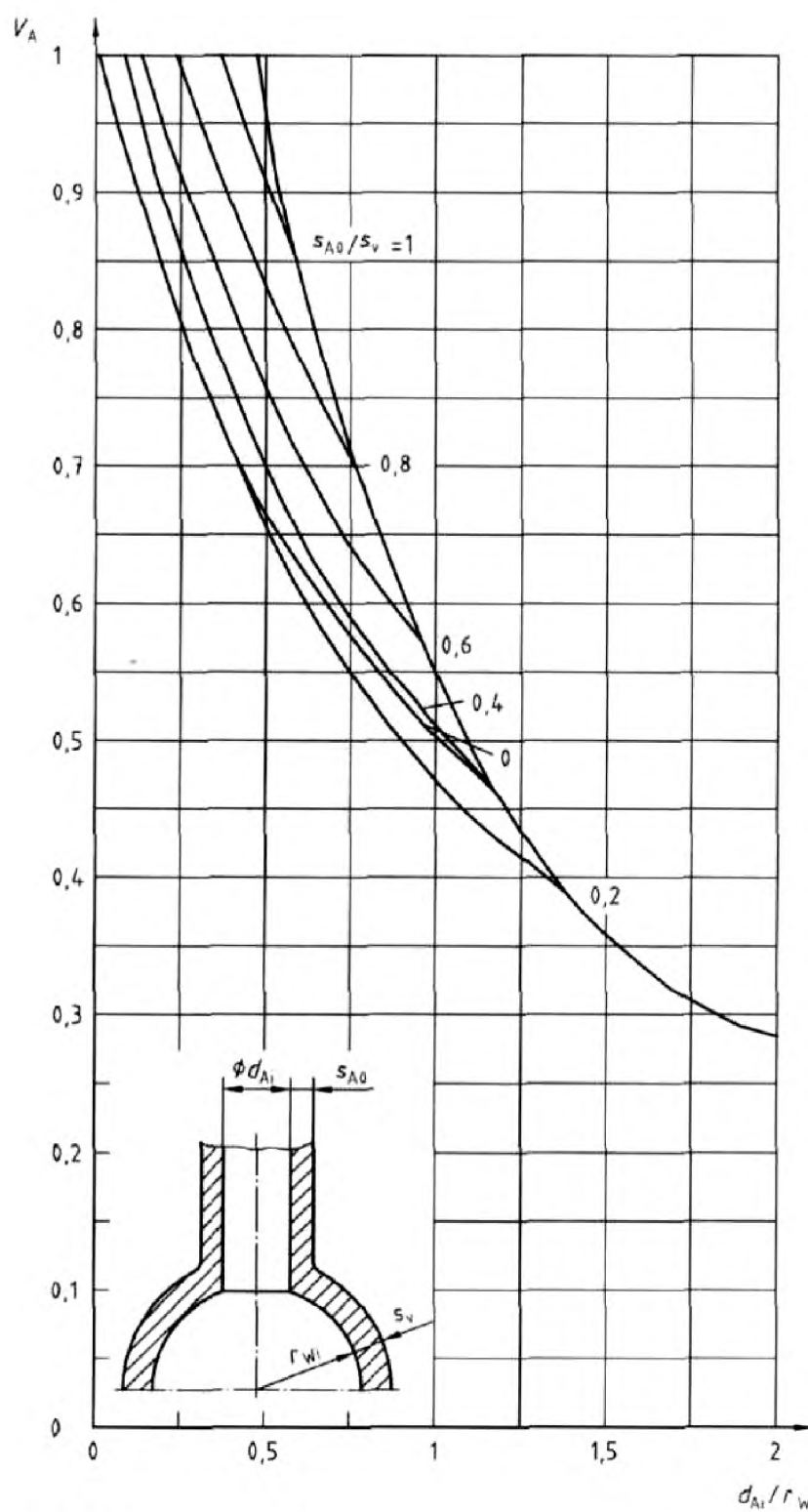
Рисунок В.16 – Значения коэффициента эффективности для сферических оболочек с вертикальным патрубком как функция d_{Ai}/r_{Wi} и s_{A0}/s_v при постоянном значении s_v/r_{Wi}
