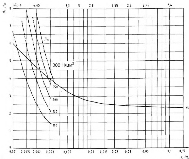
Рисунок В.17 – Значения коэффициентов формы \beta_K и \beta_{KF} для торосферических дниц
