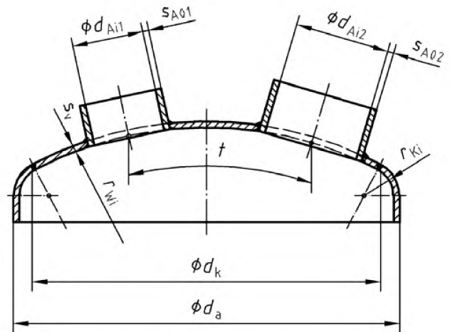
Рисунок В.2 – Выпуклое днище с отверстиями
