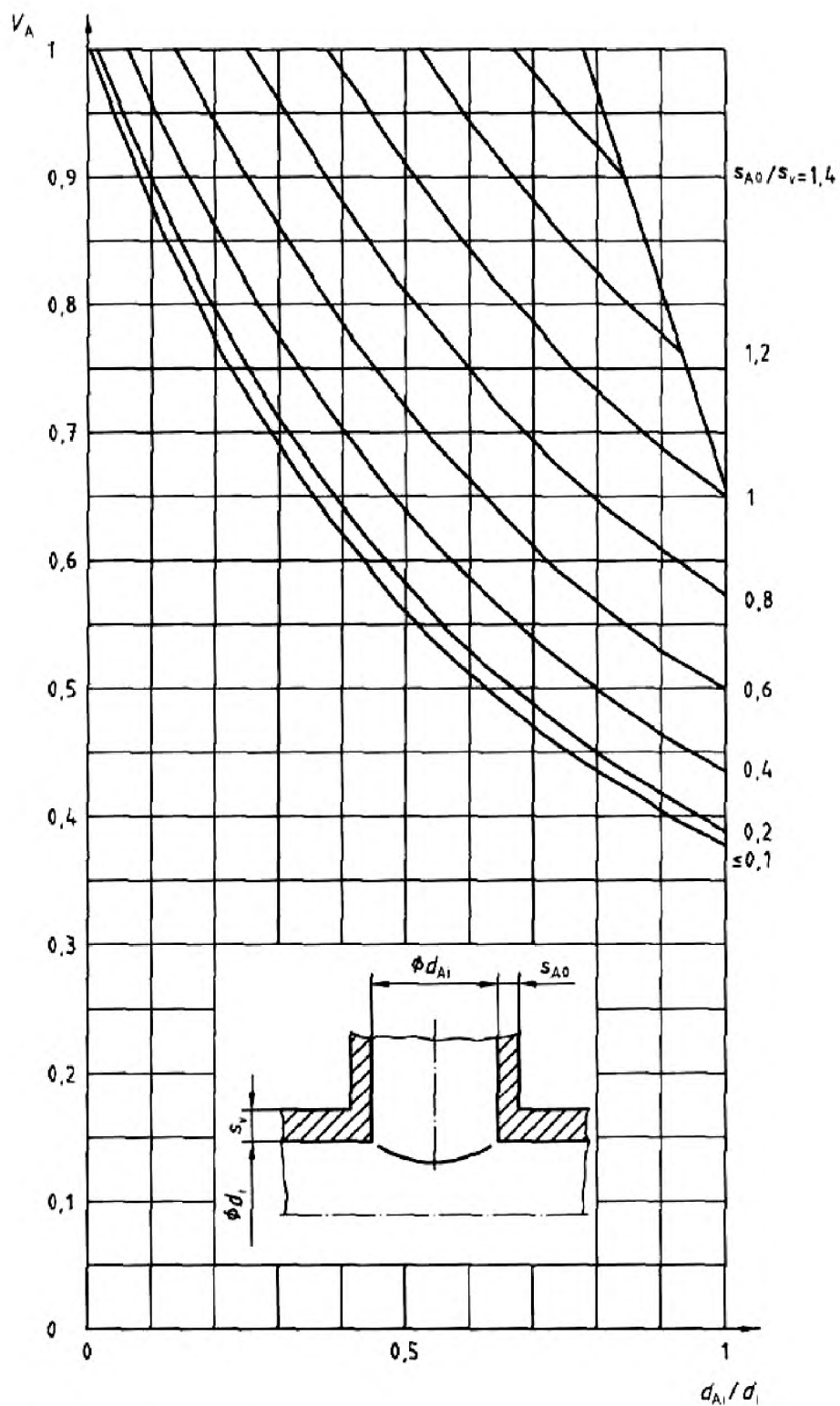
Рисунок А.23 – Коэффициент эффективности для цилиндрических обечай с вертикальным патрубком, используемый для проверки правильности расчета готовых конструкций ( s_v/d_i = 0,2 )
