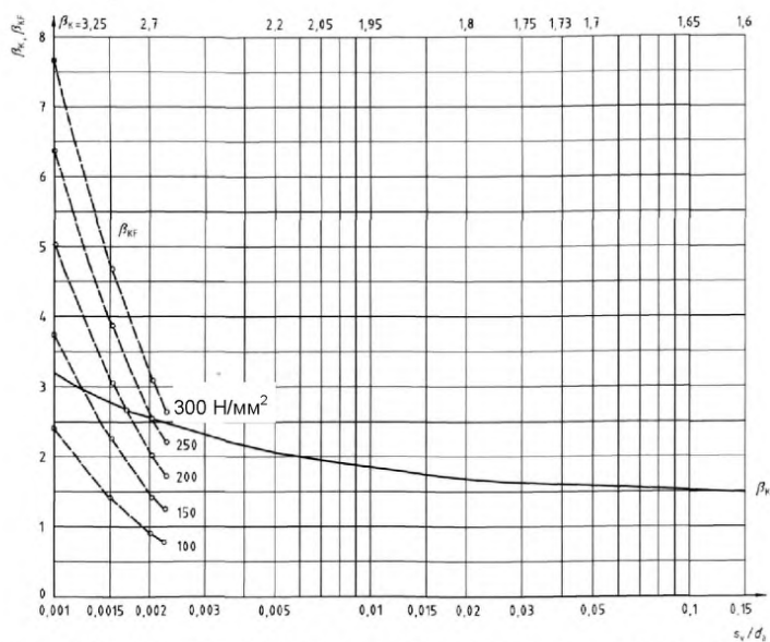
Рисунок В.18 – Значения коэффициентов формы \beta_K и \beta_{KF} для эллиптических дниц
