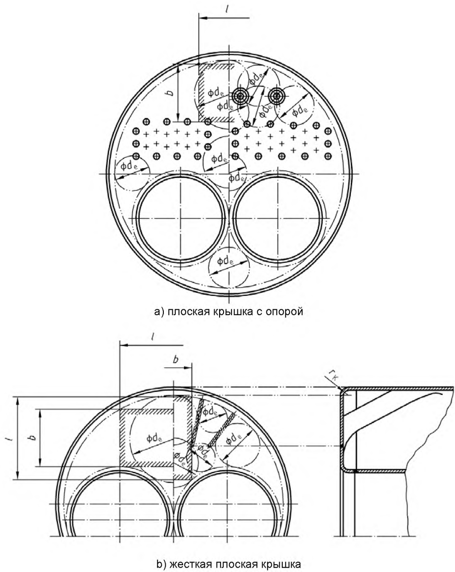
Рисунок D.8 – Плоская крышка
