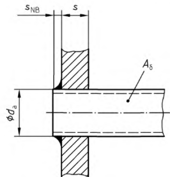
Рисунок D.13 – Вварная анкерная штанга
