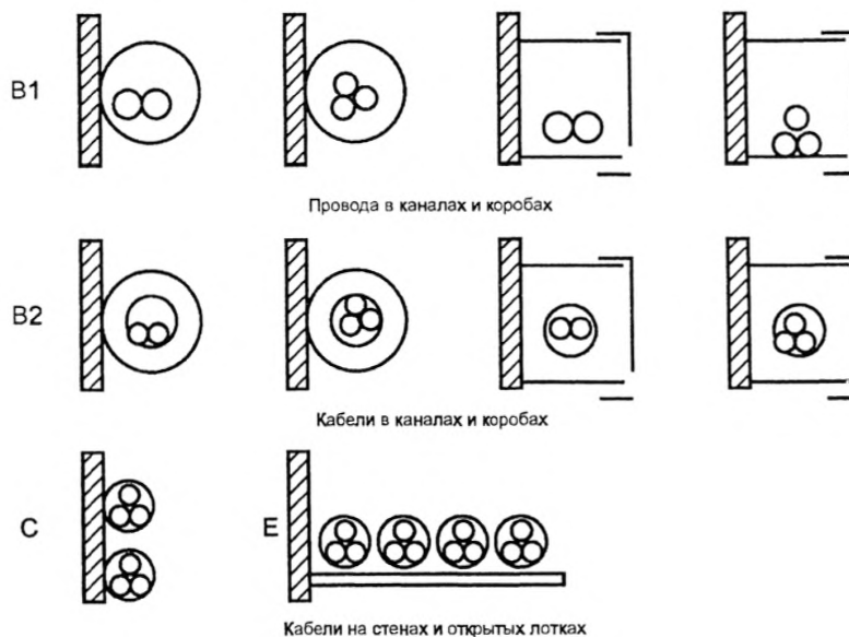
Рисунок С.1 – Методы укладки кабелей и проводов
