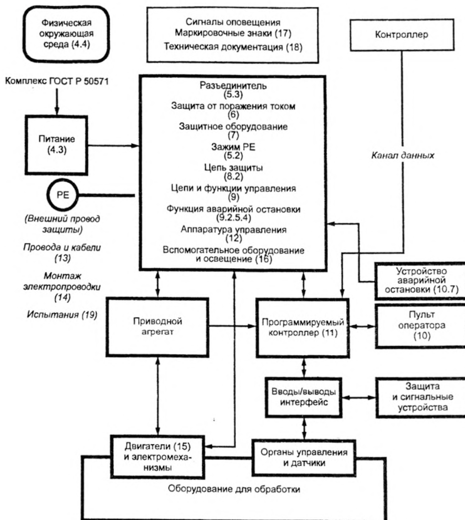
Рисунок 2 – Функциональная схема типовой машины
