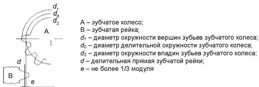
Рисунок 8 – Правильное зубчатое зацепление
