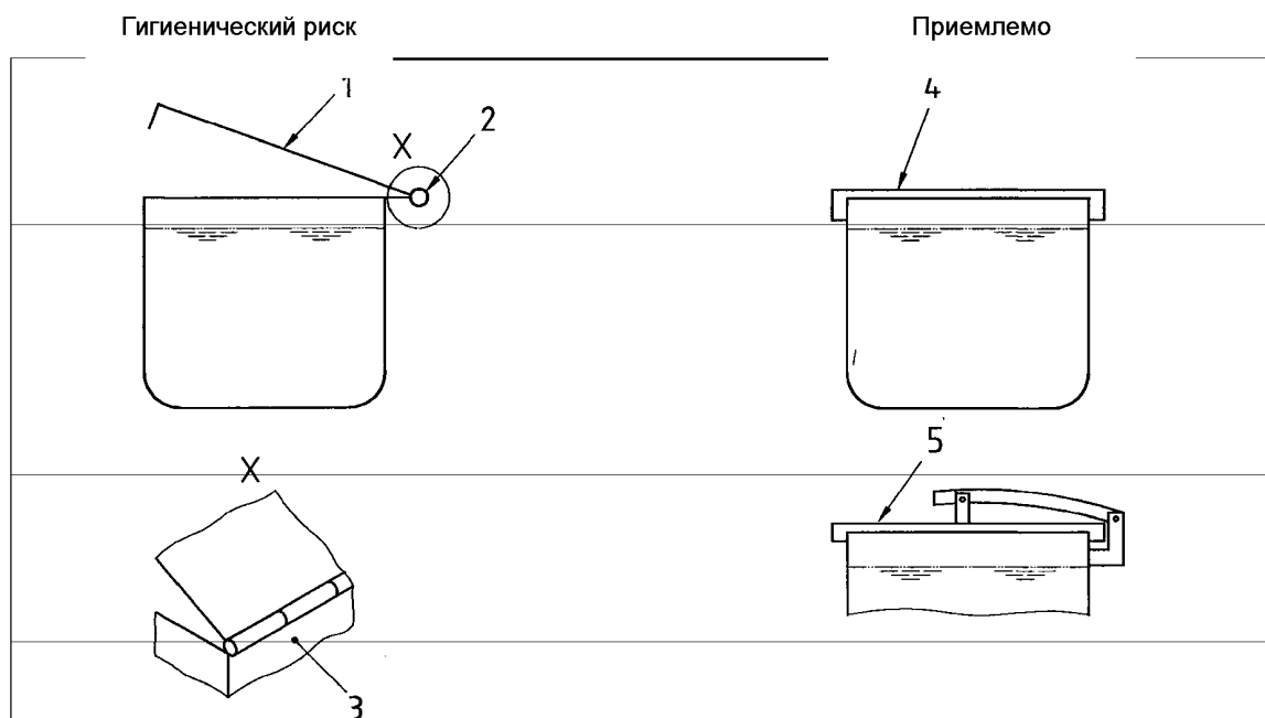
Рисунок В.11 – Проемы и крышки
