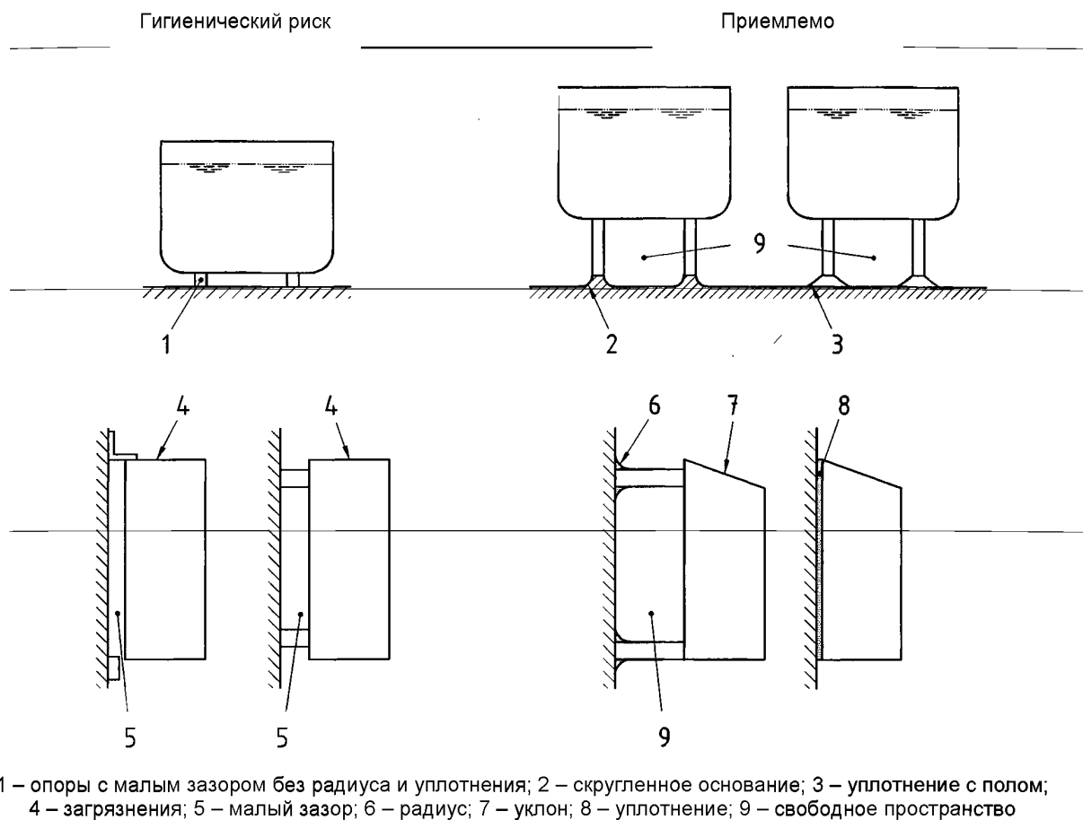
Рисунок В.13 – Крепления к полу и стене
