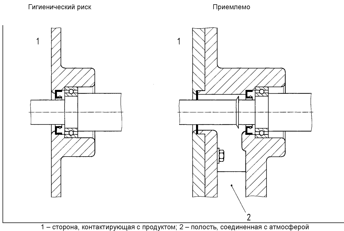
Рисунок В.9 – Конструкция входа вала
