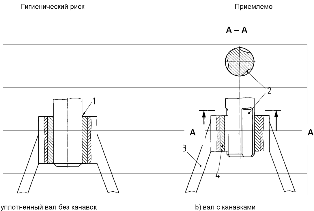
Рисунок В.9 – Конструкция входа вала
