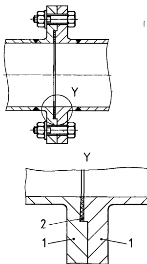
Рисунок В.5, лист 1 – Разборные соединения
