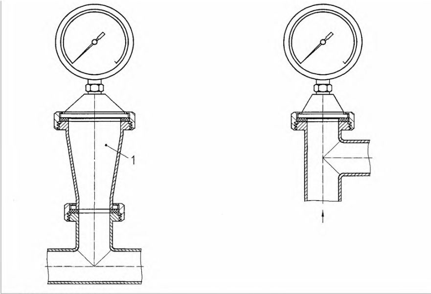
Рисунок В.3, лист 1 – Мертвая зона
