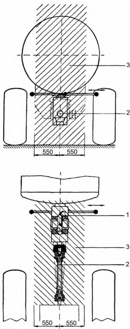
1 – компрессор или насос; 2 – ось ВОМ; 3 – пространство, в котором не должны располагаться органы ручного управления компрессором или насосом
