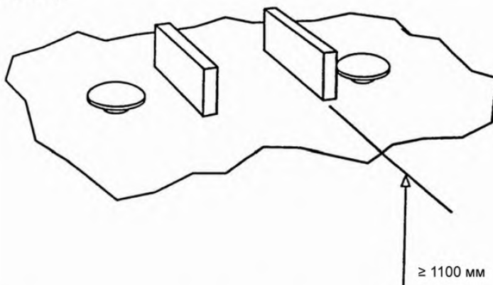
Рисунок А.11 – Предотвращение несанкционированного включения месторасположением
