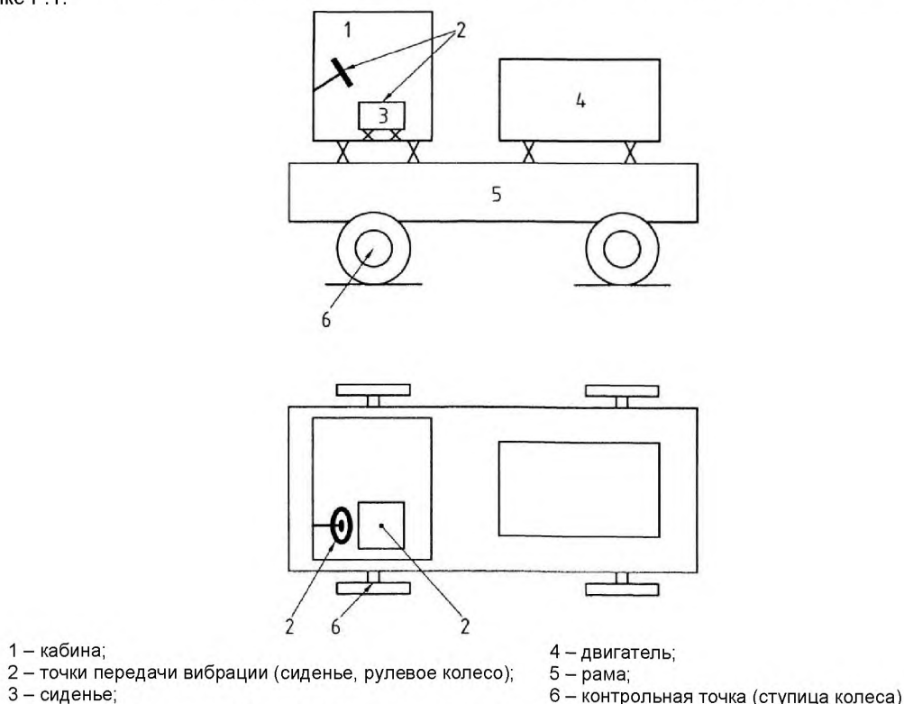
Рисунок F.1 – Пример расположения контрольной точки и точек передачи вибрации
