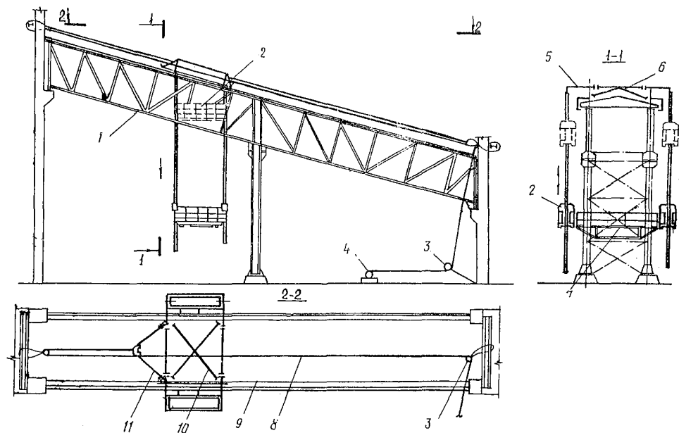
Рис. 2.12. Схема усиления транспортных галерей с помощью специального приспособления: 1 - усиливаемая конструкция; 2 - люлька; 3 - отводной блок; 4 - лебедка; 5 - консоль; 6 - съемный ригель; 7 - рабочий настил; 8 - канат лебедки; 9 - направляющие; 10 - съемная связь; 11 - двухветвевой строп
