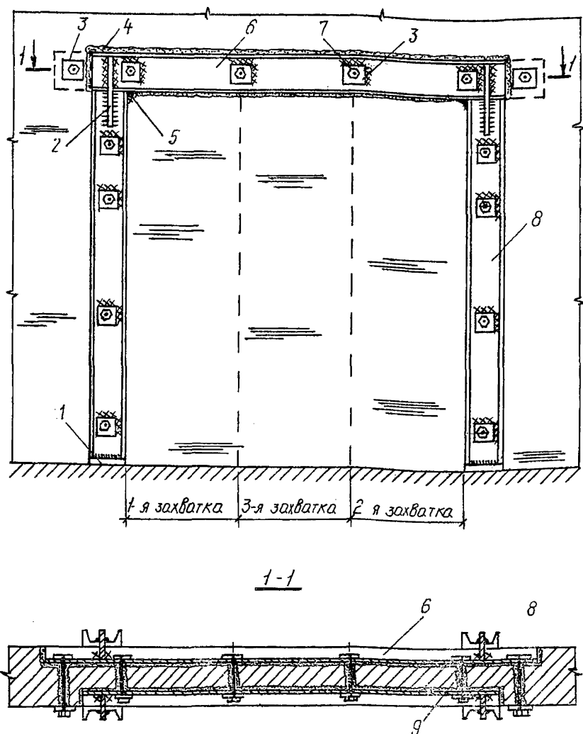
Рис. 3.10. Схема устройства временного крепления при перекладке стен и устройстве проемов: 1 - металлическая пластина; 2 - металлическая фасонка; 3 - шайба; 4 - зазор между полкой швеллера и клаской; 5 - кс- ротыш; 6 - швеллер; 7 - гайка; 8 - стойка; 9 - анкер
