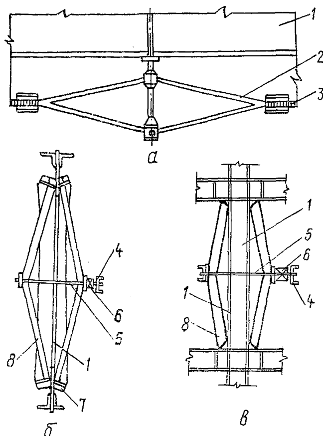
Рис. 2.5. Способы создания предварительного напряжения при усилении конструкций: а - балочных конструкций с помощью натяжного параллелограмма; б - стержней ферм; в - средних спар; 1 - существующая конструкция; 2 - натяжной параллелограмм; 3 - затяжка; 4 - траверсы; 5 - тяги; 6 - домкрат или винтовое устройство; 7 - упор; 8 - элемент усиления
