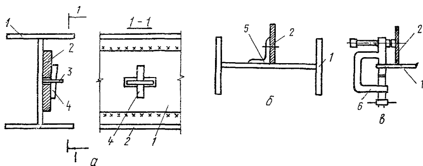
Рис. 2.1. Приспособления для сборки и выверки конструкций усиления:
