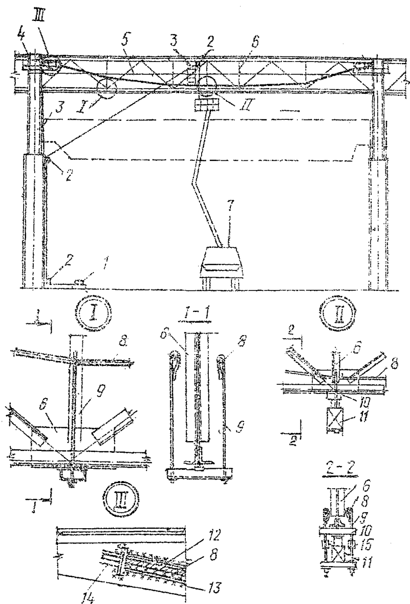
Рис. 2.13. Схема усиления ферм предварительно-напряженными затяжками:
