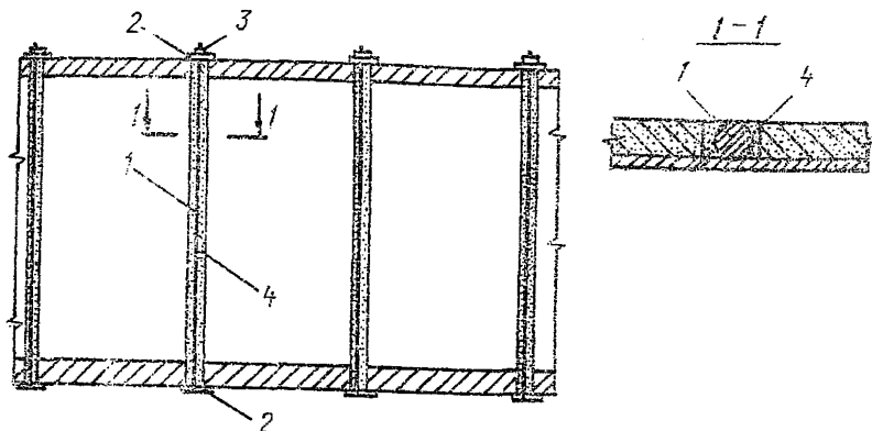
Рис. 3.4. Схема усиления каменных стен предварительно-напряженными тяжами: 1 – тяж; 2 – шайба; 3 – гайка; 4 – штраба, заполненная цементным раствором состава 1:2;
