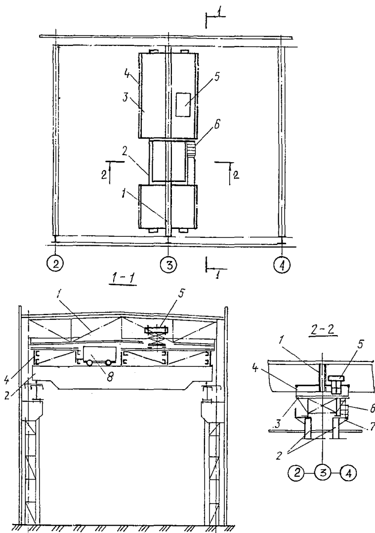
Рис. 2.II. Схема усиления ферм с мостовых кранов: 1 - усиливаемая ферма; 2 - мостовой кран; 3 - рабочий настил; 4 - съемные элементы ограждения; 5 - инвентарные под- мости; 6 - лестница; 7 - рабочий настил с ограждением; 8 - те- лезка крана
