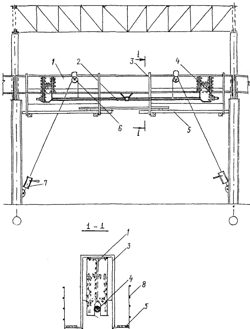
Рис. 2.16. Схема усиления балок предварительно-напряженными затыжками: 1 - усиливаемая конструкция; 2 - затыжка; 3 - кронштейн; 4 - натяжное устройство; 5 - настил; 6 - отводной блок; 7 - лебедка; 8 - элементы ограждения
