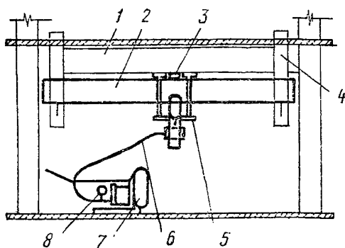
Рис. 2.7. Схема включения в работу балочных конструкций: 1 - усиливаемая балка; 2 - балка усиления; 3 - прокладка; 4 - хомуты; 5 - захватно-натяжное устройство с упорами; 6 - шланг; 7 - масляная станция; 8 - динамометр
