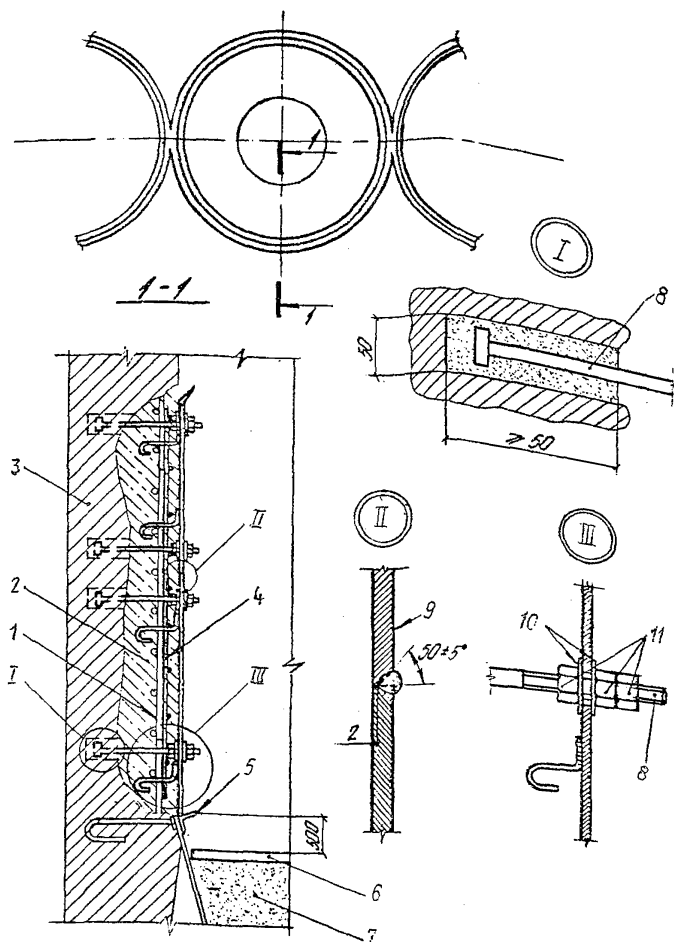
Рис. 1.15. Схема местного усиления стенки силоса:
