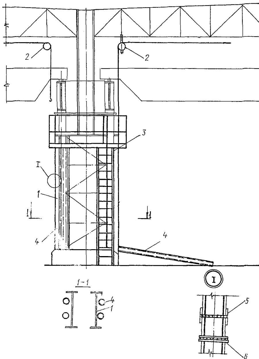
Рис. 2.9. Схема усиления колонн дополнительными элементами, напрягаемыми в заводских условиях: I - усиливаемая колонна; 2 - отводные блоки; 3 - лестница с площадкой; 4 - элементы усиления; 5 - элементы соединения наружных труб; 6 - торцовые детали
