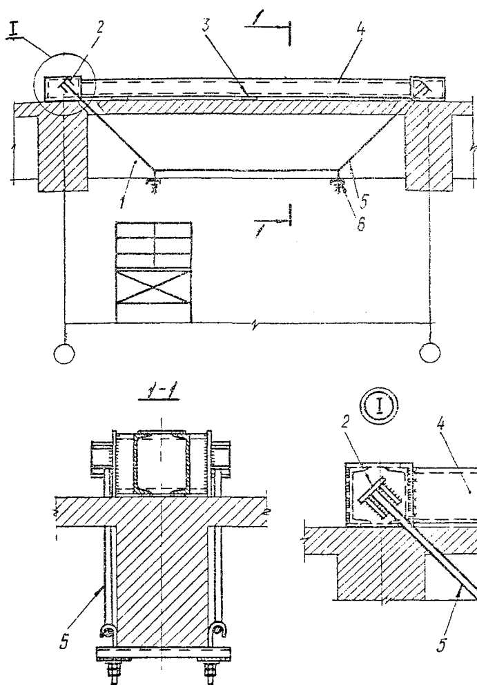
Рис. I.I0. Схема усиления балки шпренгельной затяжкой с закреплением на металлическую балку: I - усиливаемая балка (ригель); 2 - анкерное устройство; 3 - подкладка; 4 - балка усиления; 5 - шпренгельная затяжка; 6 - тяж
