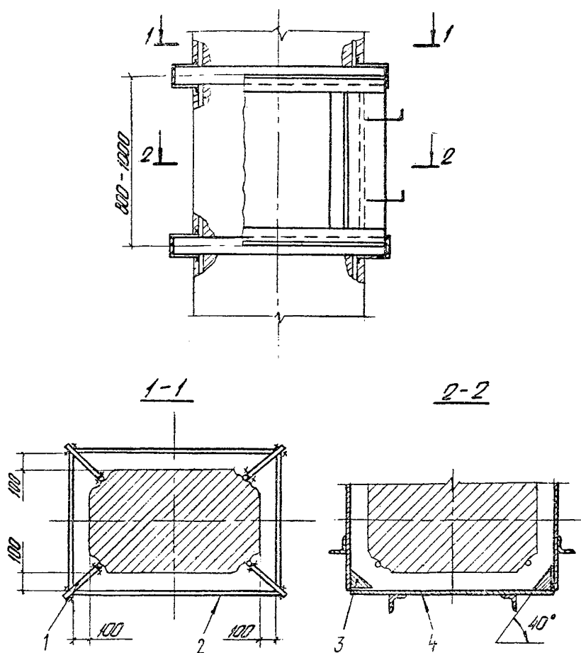
Рис. I.4. Схема крепления щитов опалубки к обоямам: 1 - планка; 2 - пластины воротника; 3 - фаскообразователь; 4 - щит опалубки
