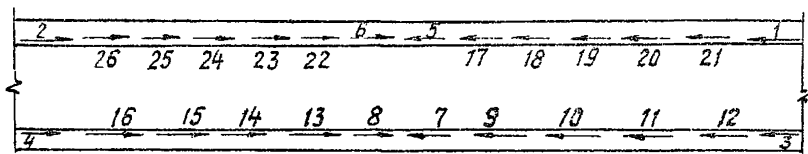
Рис. 2.3. Порядок наложения швов (1–26) при усилении длиномерных элементов
