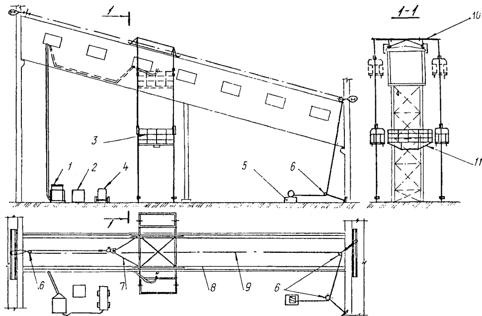
Рис. 1.17. Схема усиления железобетонных стен галерей: 1 - торкрет-установка; 2 - контейнер для сухой бетонной смеси; 3 - льюшка строительная; 4 - компрессор; 5 - электролебедка; 6 - отводной блок; 7 - двухветевой строп; 8 - направляющие; 9 - канат лебедки; 10 - сазаки; 11 - рабочий настил
