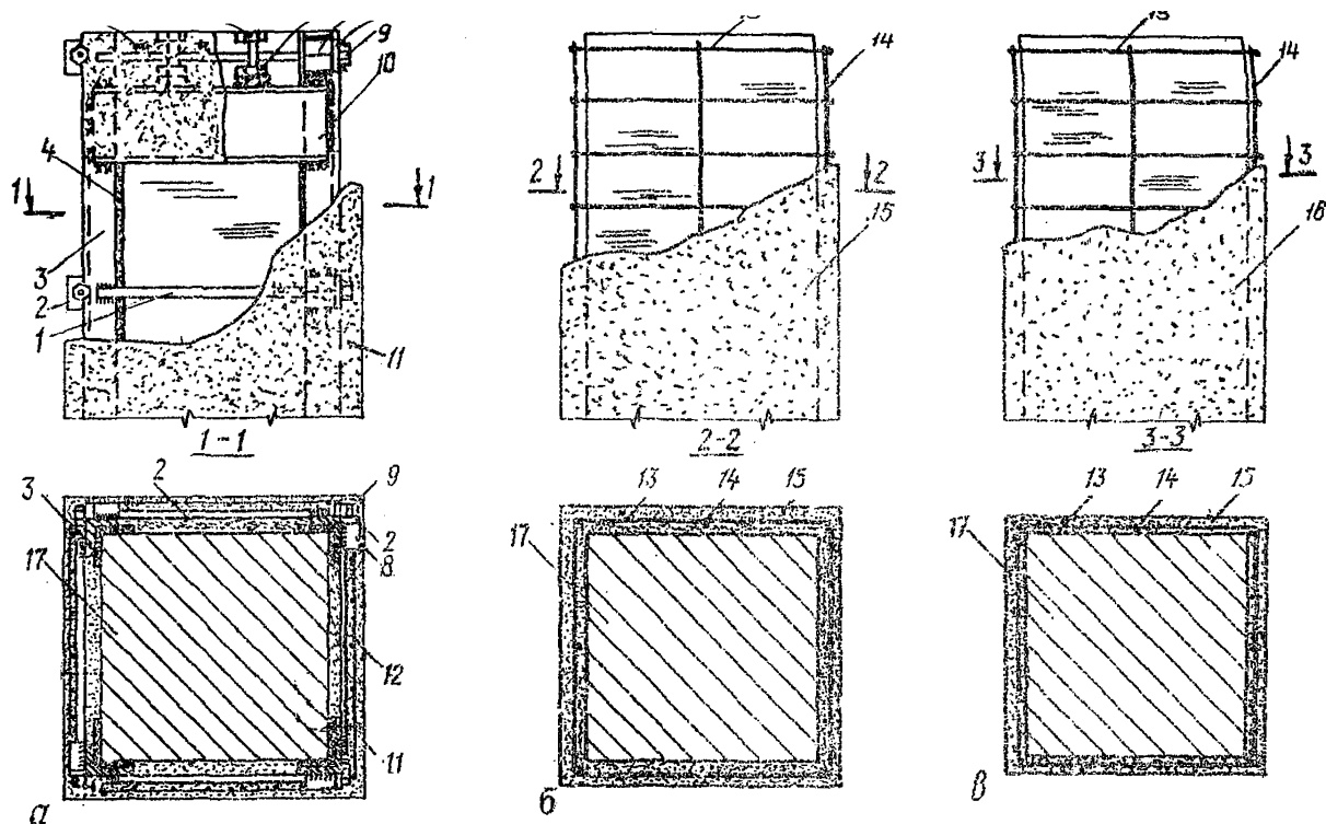
Рис. 3.7. Схема усиления каменных простенков и столбов обоймами:
