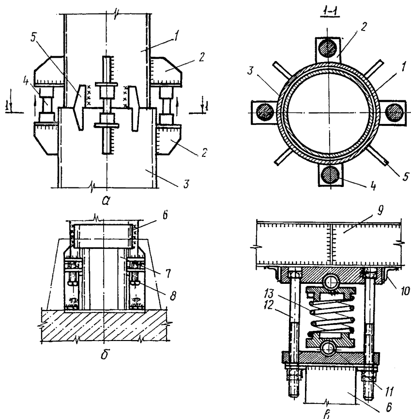
Рис. 2.6. Способы включения в работу дополнительных опор: а - раздвижной телескопической стойки; б - выжиманием с помощью винтовых приспособлений; в - специальной установкой; г - внутренней трубой; 2 - упоры; 3 - наружная труба; 4 - домкраты; 5 - направляющие ребра; 6 - подводящая опора; 7 - усиливаемая колонна; 8 - натяжные болты; 9 - усиливаемая балочная конструкция; 10 - фиксаторы; 11 - шаровые опоры; 12 - регулирующие стяжные болты; 13 - пружина
