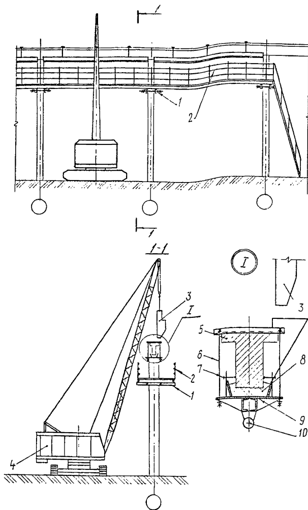
Рис. I.9. Схема усиления подкрановой балки с креплением рабочих площадок на металлических консолях: I — металлическая консоль; 2 — рабочая площадка с ограждением; 3 — бадья для бетона; 4 — монтажный кран; 5 — уси- ваемая балка; 6 — подвеска; 7 — прижимной винт; 8 — бетон уси- ления; 9 — блок-форма; 10 — вибратор
