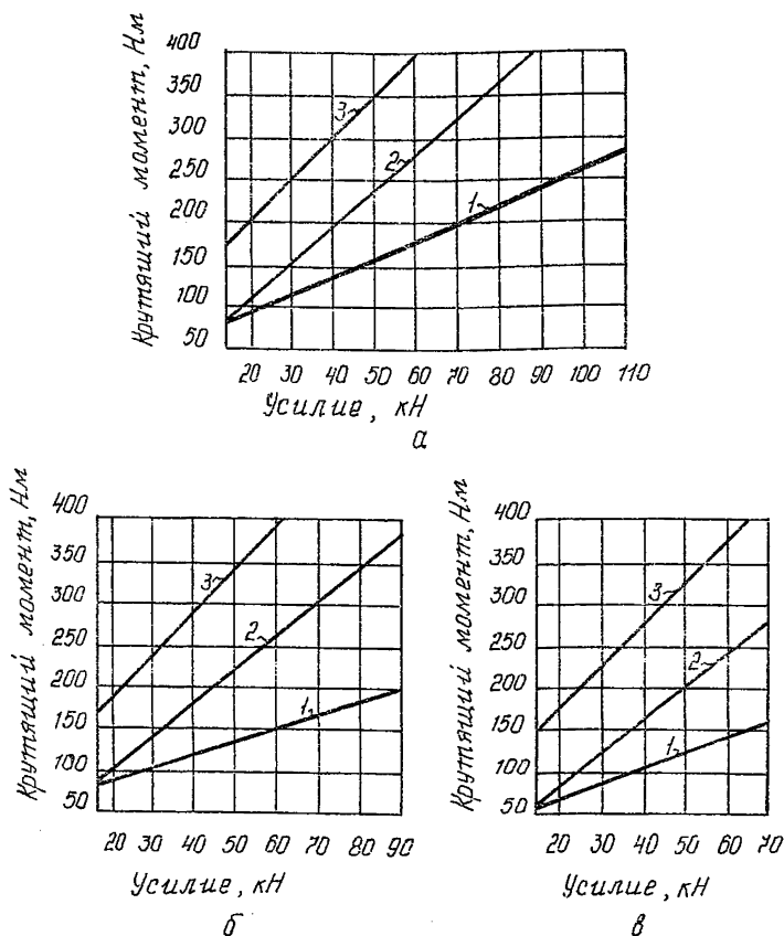
Рис. 3.3. Графики зависимости "крутящий момент - усилие": а - для болтов \varnothing 25 мм, тип резьбы M24x3; б - для болтов \varnothing 22 мм, тип резьбы M22x3; в - для болтов \varnothing 20 мм, тип резьбы M20x2,5; 1 - при полном отсутствии момента трения на контакте торцовых поверхностей; 2 - при чистых сухих поверхностях контакта; 3 - при грязных поверхностях контакта
