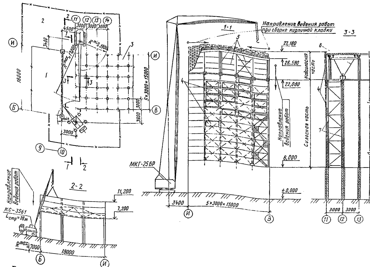
Рис. 1.18. Схема усиления и восстановления строительных конструкций комбикормового завода:
