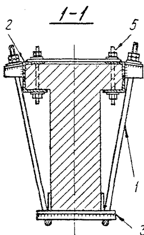
Рис. 1,12. Схема усиления подкрановых балок шпренгельной затяжкой с креплением к обойме полки: I - шпренгельная затяжка; 2 - обойма полки; 3 - центрирующие подкладки; 4 - анкерное устройство; 5 - шпилька обоймы
