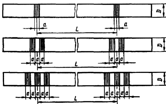
Рисунок 1. Ширина предупреждающих колец и расстояние между ними
