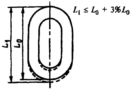
Рисунок 1 Увеличение звена цепи:
