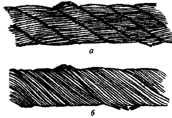
Рисунок 2. Сочетание обрывов проволок с их износом:
