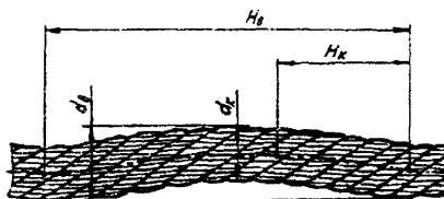
Рисунок 9. Волнистость каната
