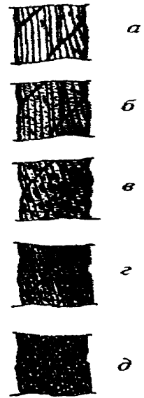
Рисунок 6. Поверхностная коррозия проволок каната крестовой свивки:
