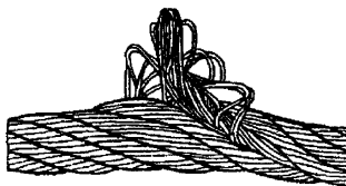
Рисунок 11. Выдавливание сердечника
