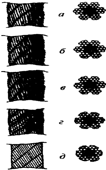
Рисунок 5. Износ наружных проволок каната крестовой свивки:
