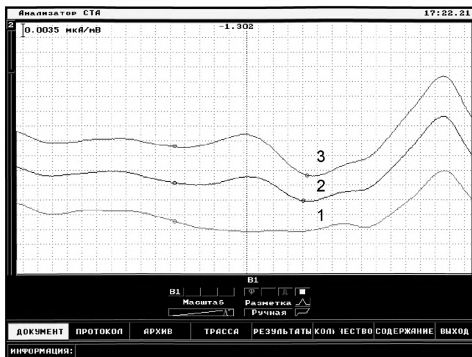
Рисунок 2. Вольтамперограмма определения витамина B_2 в растворе фонового электролита (1), в пробе (2) и в пробе с добавкой стандартного раствора
