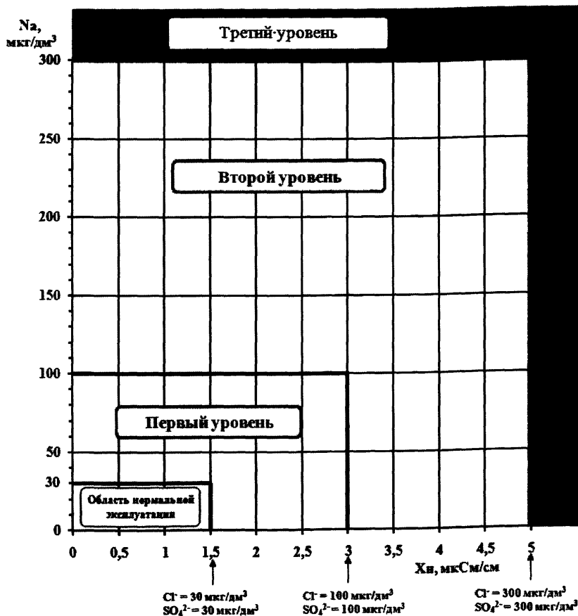
Рисунок Б.2 – Уровни отклонений нормируемых показателей качества продувочной воды ПГ при эксплуатации энергоблока на уровнях мощности \geq 50\% N_{ном}
